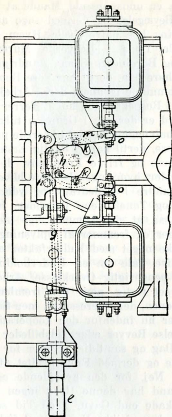
Fig. 2. Det ene Gliderpar set udvendigt fra.
