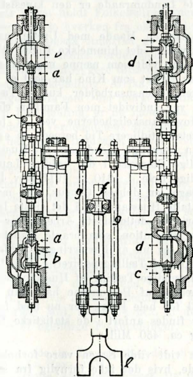
Fig. 1. Dampcylinder med fire Glidere.
