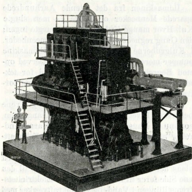
Fig. 1. Model af en 5700 H. K. Stempeldampmaskine for 100 at Damptryk. De cylindriske Beholdere ved højre Side er Mellemoverhedere.
