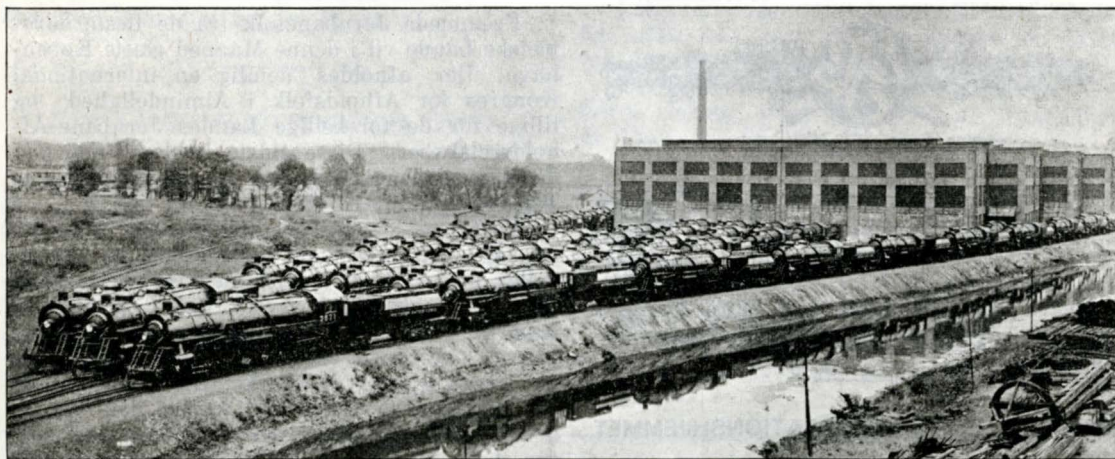
Fig. 1. 50 1 E 1 Lokomotiver til „Southern Pacific“ Jernbanen samlede og færdige til at forlade Baldwin's Lokomotiv Værksted.
