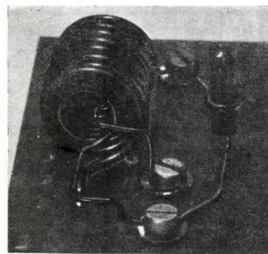
Opbygningen af transformer-spolerne S1/S2.
