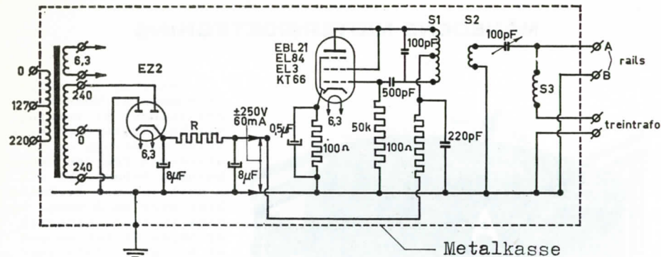
Strømskema for højfrekvens-generator.
