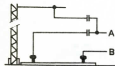
Tilslutning ved 2-skinne, jævnstrøm
