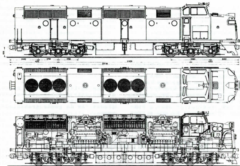
Tegning af Krauses-Maffei's 4000 hk diesellok
