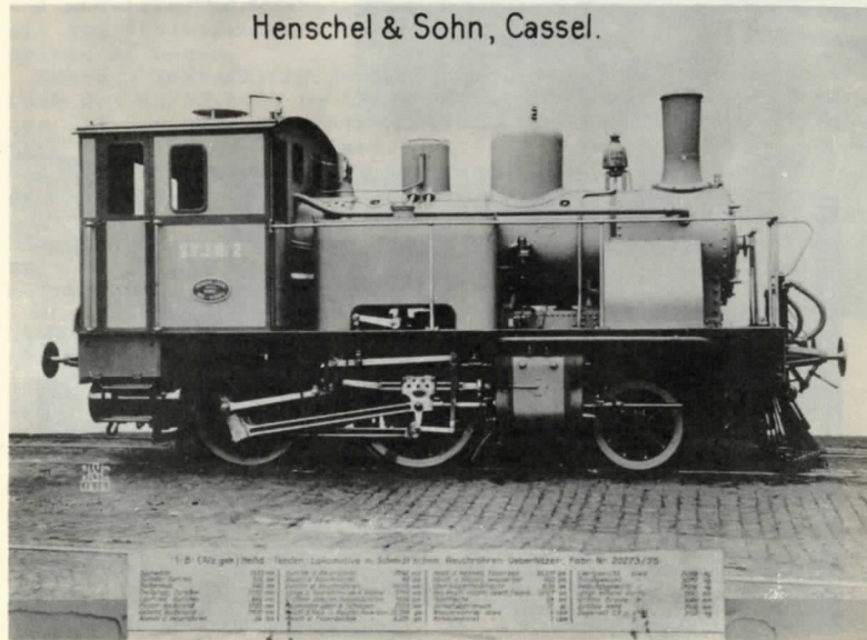
Fabrikfoto af SVJ's lok. nr. 2
