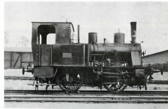
LJ's nr.23 i Hillerød, også solgt til stålvalseværket. (Henschel nr.21452 - bygget 1929) Foto: Sv.J.
