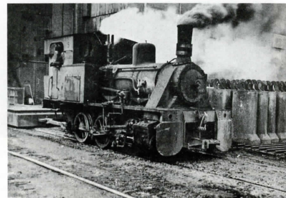
Gribskovbanens gamle "MAREN" på stålvalseværket. Foto: Sv.J.
