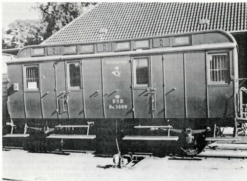
Batterispændingen til vognens egenbelysning er 32 volt. Vognen kan sammenkobles med ltr. DL, D0 og DP til dobbeltpost-
