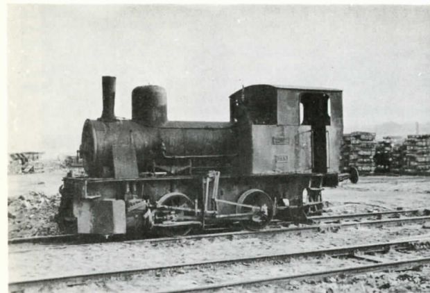
"DAN" fra Hedehusenes skærvefabrik, nu i Frederiksværk. (Henschel nr.10564 - bygget 1911). Foto: Sv.J.
