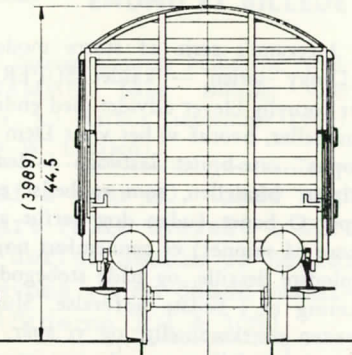
lukket UIC standardvogn
