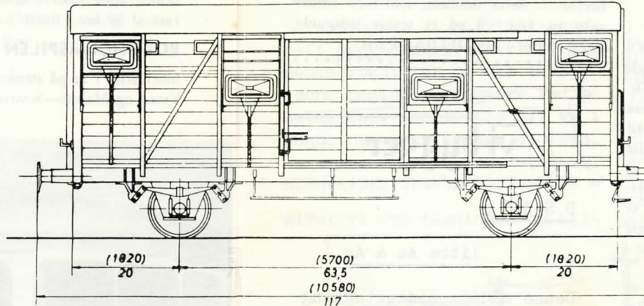
lukket UIC standardvogn
