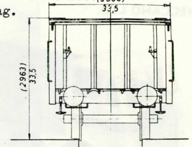
åben UIC standardvogn
