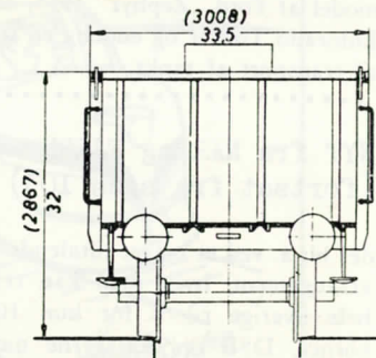
åben UIC standardvogn
