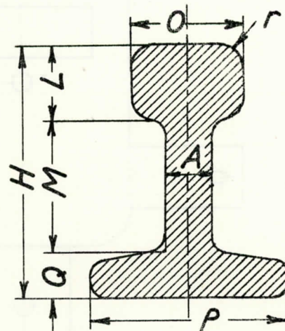
Modelskinneprofil
