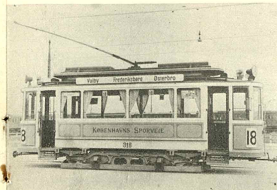
Fig. nr. 1. Første under kommunen bygget motorvognstype.
