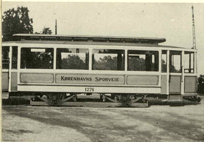
Fig. nr. 7. Langsædet bivogn med ombyggede, lukkede perroner. (Fot. Jan Walter.)
