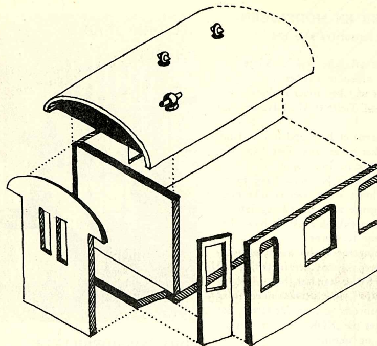
Axonometri visende vognkassens samling
