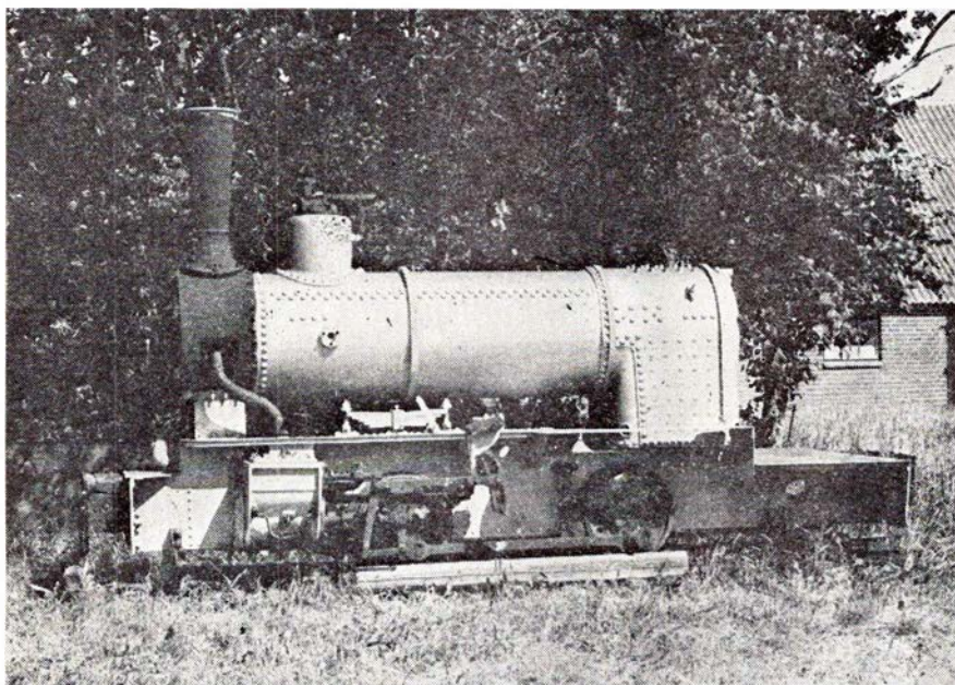
Lars Andersens Henschel-lokomotiv (17819/1921) under restaureringen, til hvilken han fik kr. 2.500 af »Støtteforeningen Danske Dampvenner«. Foto: Lars Andersen.
