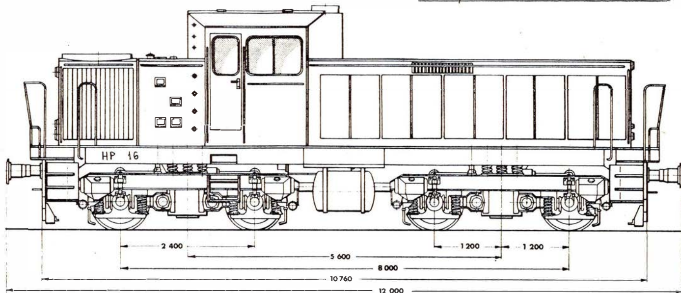
Dieselhydraulisk lokomotiv - HENSCHEL DHG 1200
