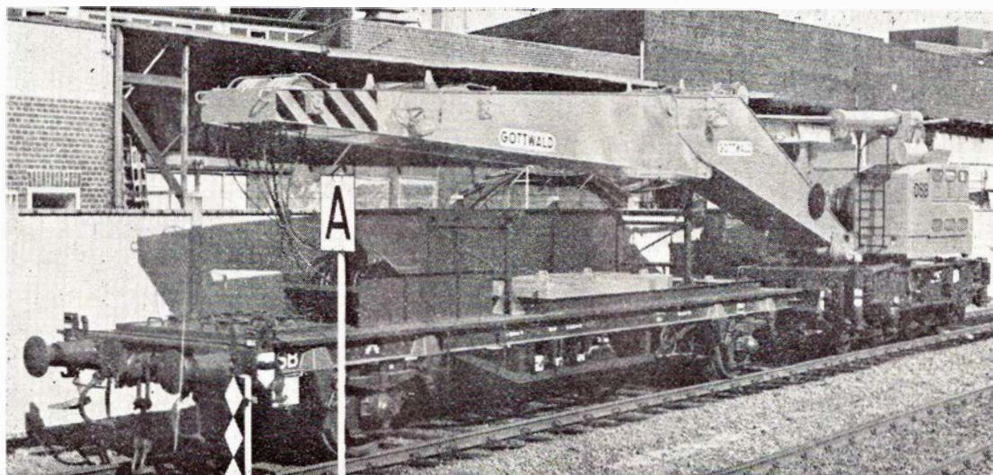
25 tons sporrægningskran, fabrikat GOTTWALD, leveret i juli 1976 til DSB
