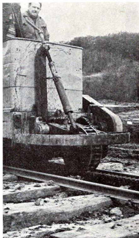
Nagbøl traktor med vippearms og skruespindel.
