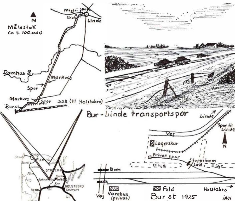
Strækingsplan for Bur—Linde sidespor
