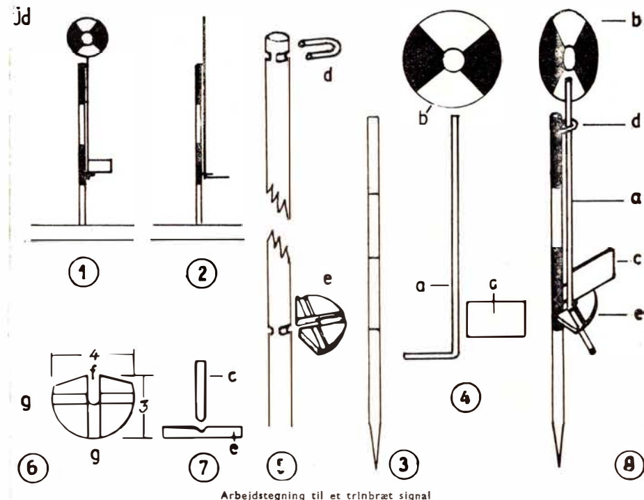
Arbejdstegning til et trinbræt signal
