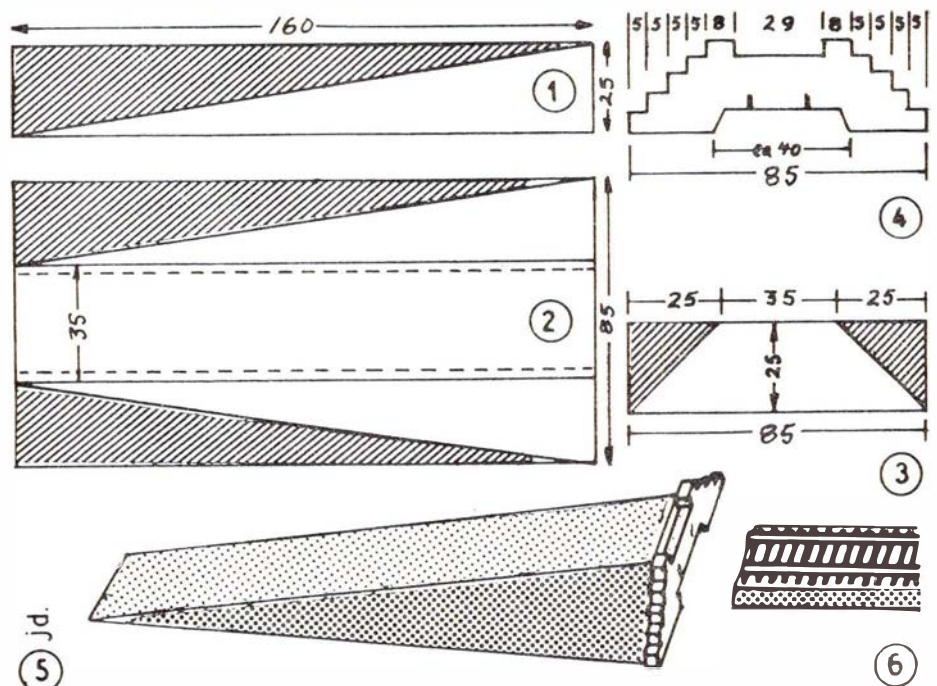
Arbejdstegning til en enderampe
