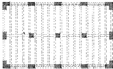
FUNDAMENTSPLAN NO 2.
