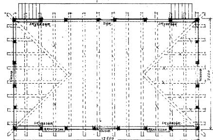
PLAN AF VAREHUSET
