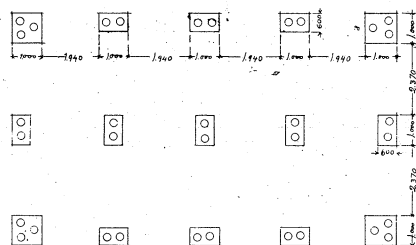
FUNDAMENTSPLAN NO 1.
