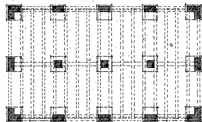
FUNDAMENTPLAN.
