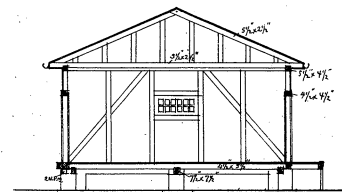
KORTSNIT
