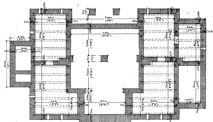
FUNDAMENTPLAN.
