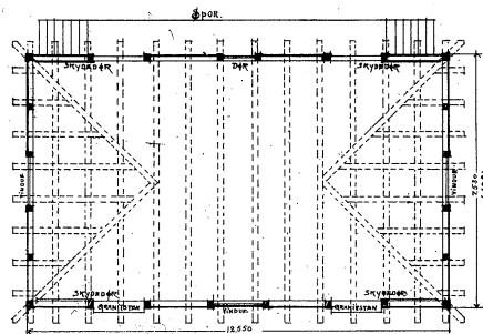
STUEPLAN
