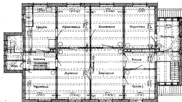
1 ste PLAN.
