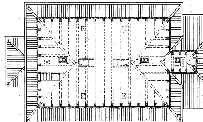
LOFTPLAN.
