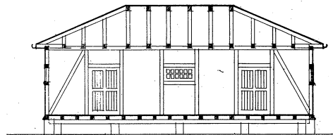
LANGSNIT
