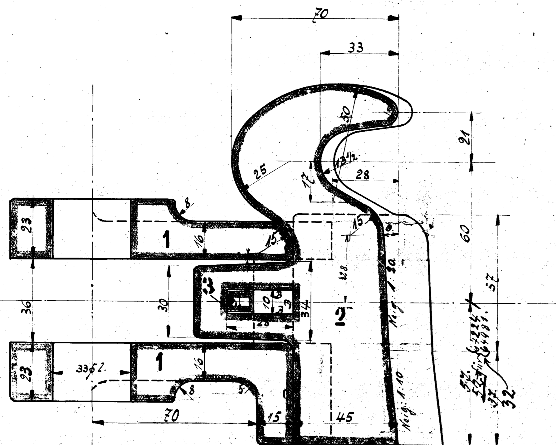
Schnitt A-B Aussen
