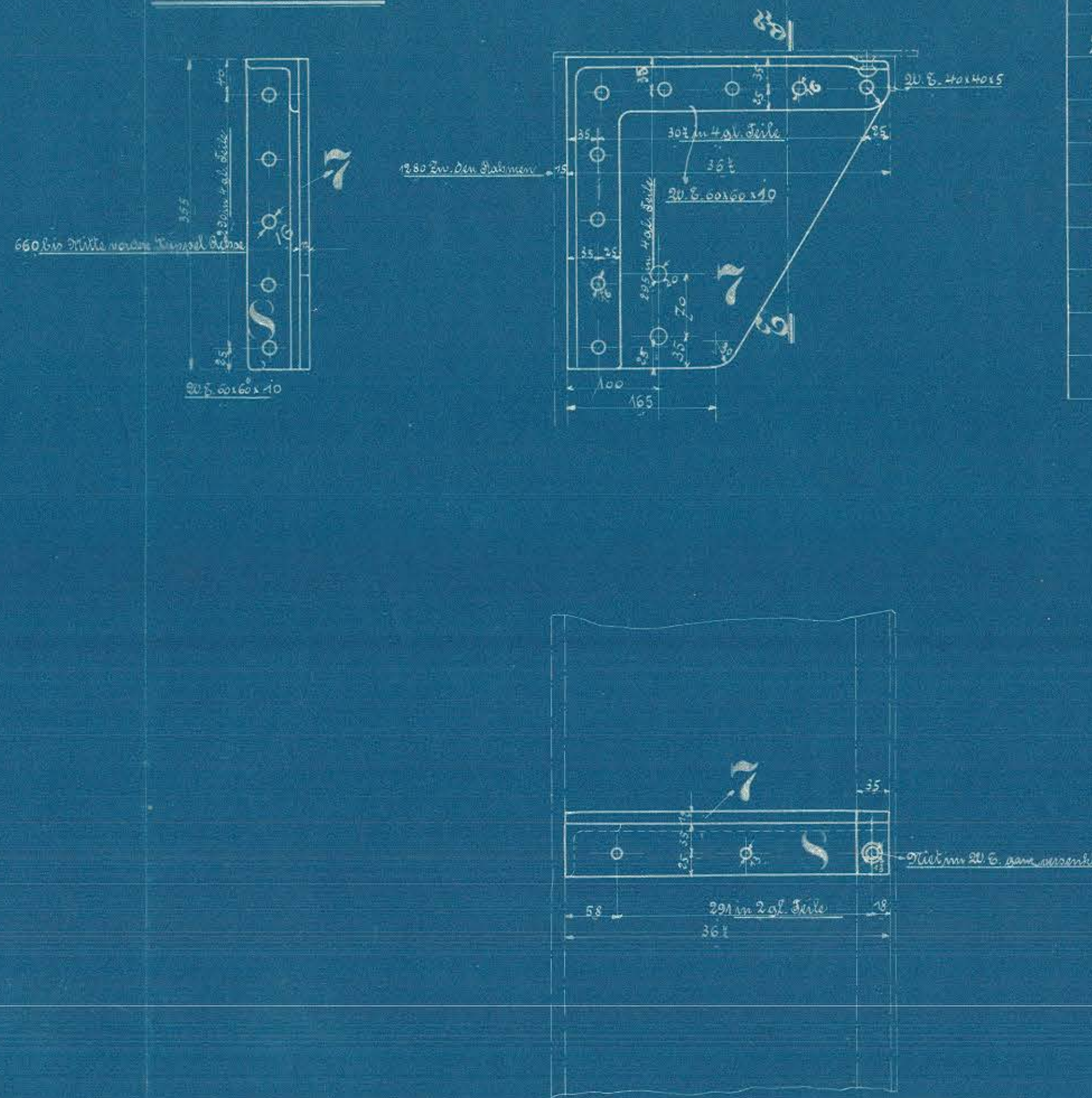
Schnitt E-F
