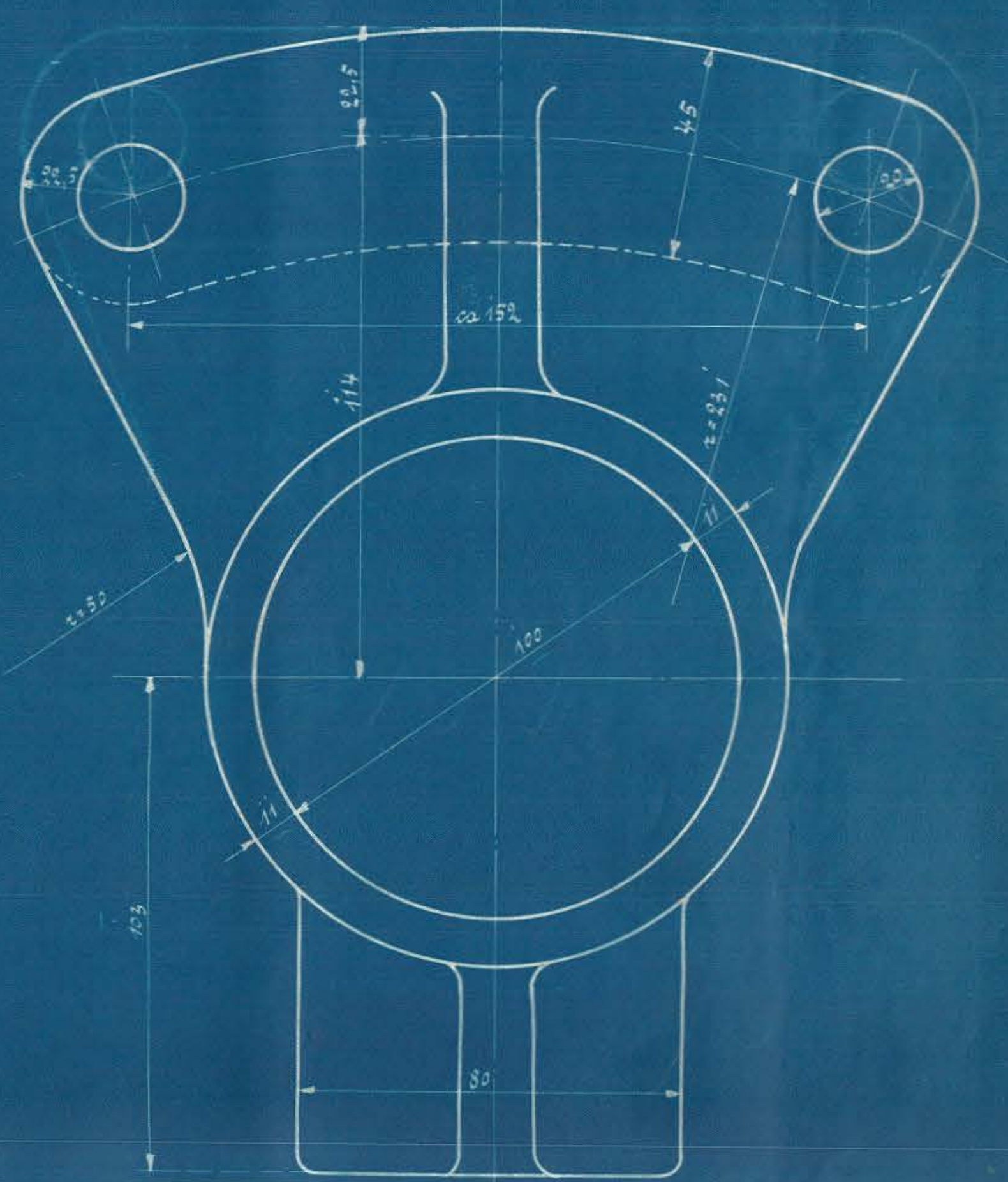
Regulator - Stimmscheibe zu den 10 Dampf-Lampfen-Schematen für die Ostjællandske Eisenbahn, Hjørslev. Tab. 10 10031-32
