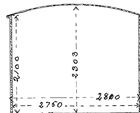
Snit G-H.
