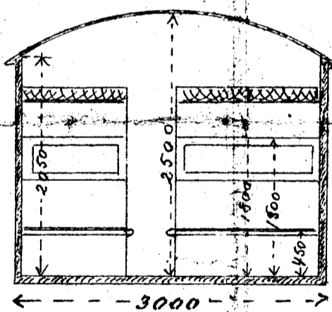
Snit C-D.
