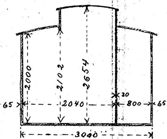
Snit A-B.
