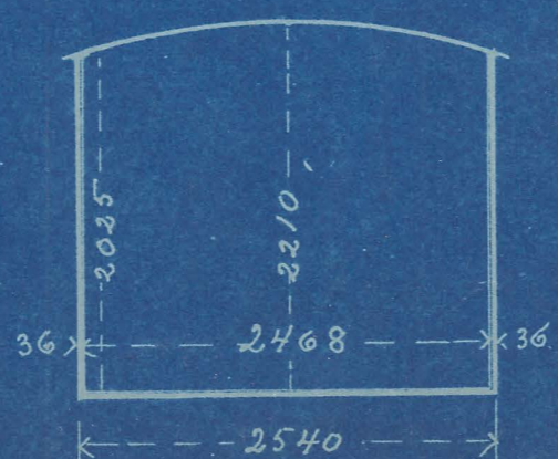
Snit I-L
