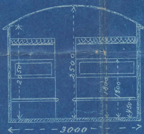
Snit C-D.
