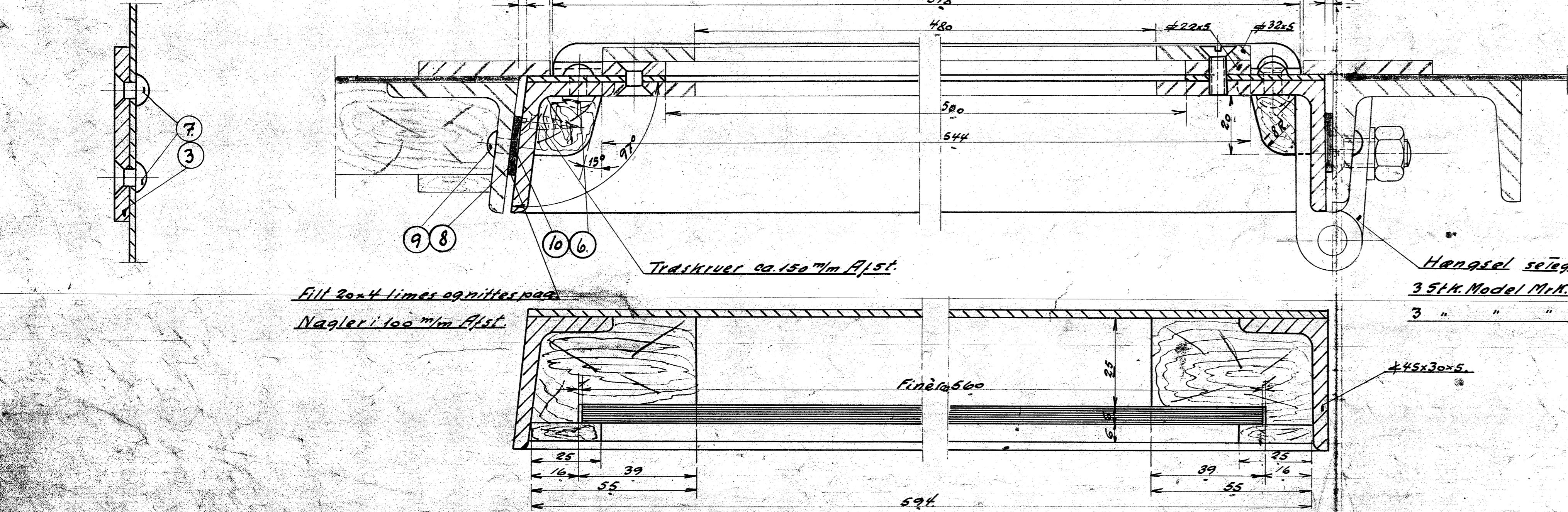
Snit A-A
