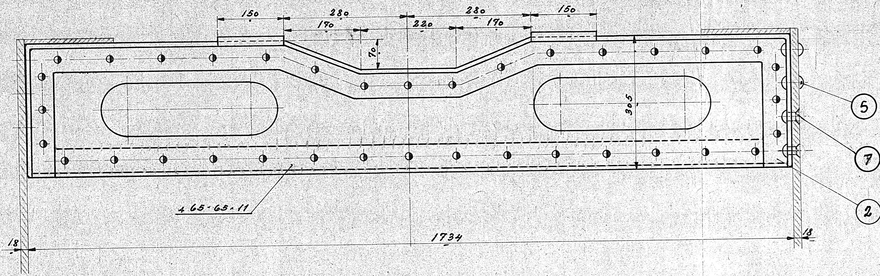
Fundamentplade. Teg. 120 L-8.19.
