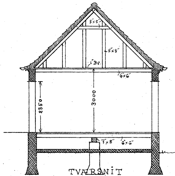
TVÆRSNIT
