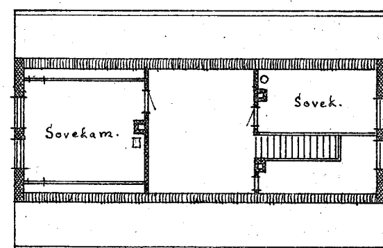
1:1200 TAGPLAN.
