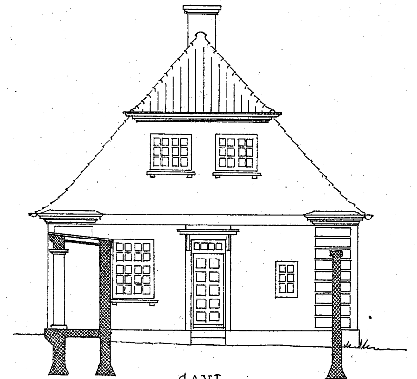
GAVL.
