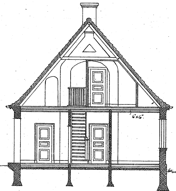
SNIT A-B.
