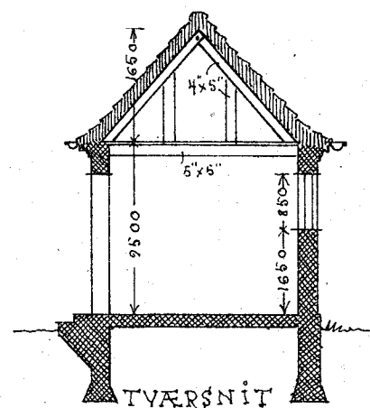
TVÆRSNIT
