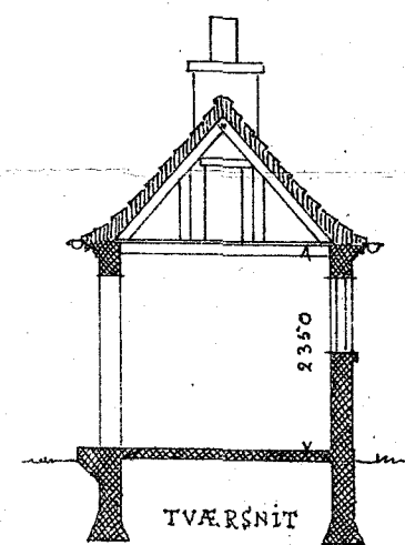
TVÆRSNIT
