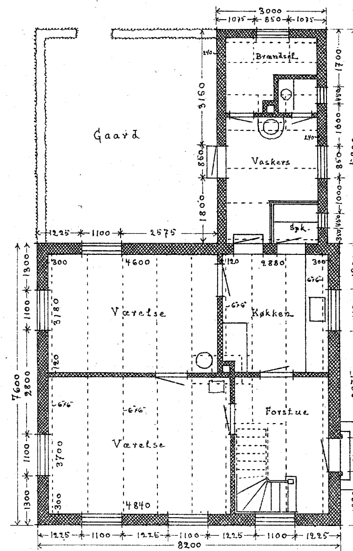
STUEPLAN
