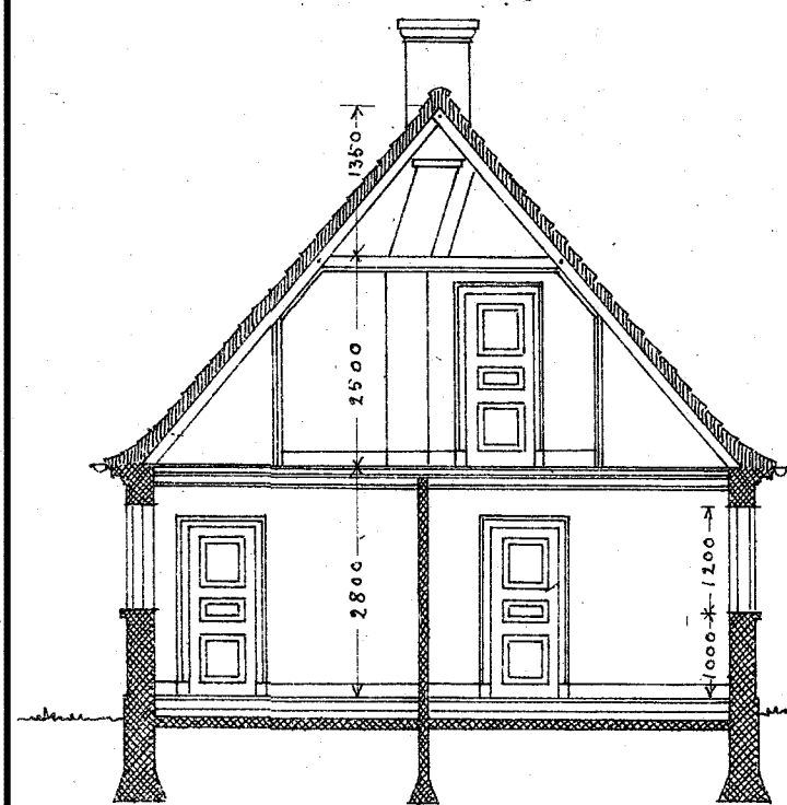
TVÆRSNIT
