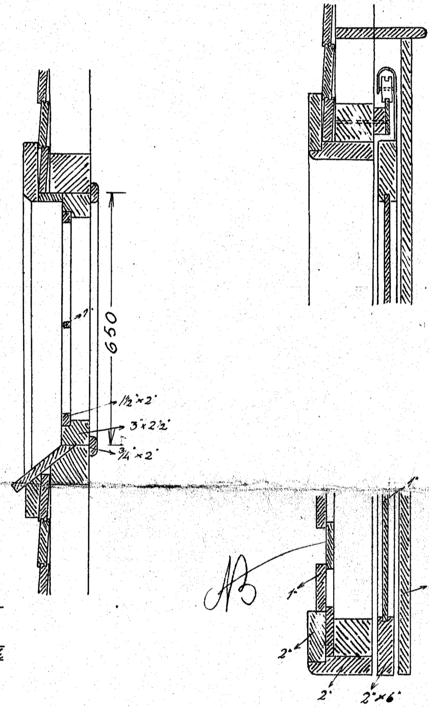
Tværsnit.
