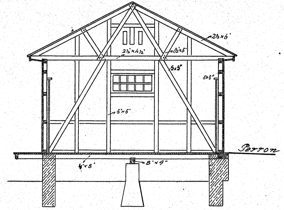
Tværsnit.
