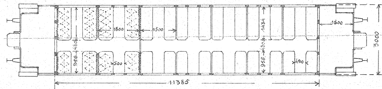
Bagagevogn.
