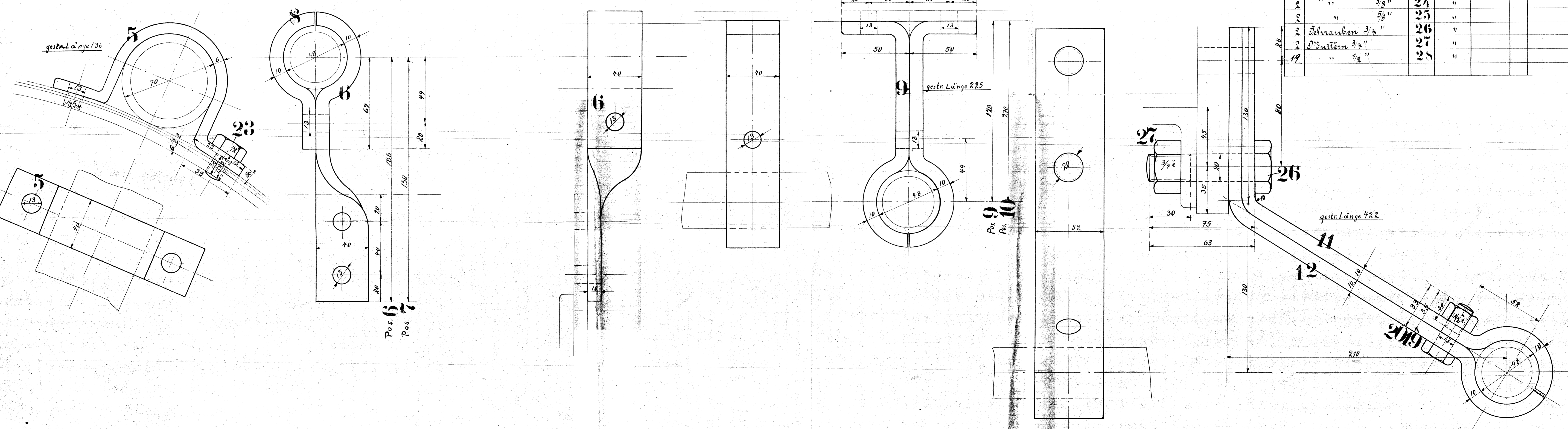
Stahrschellen & Bremsleitung.
