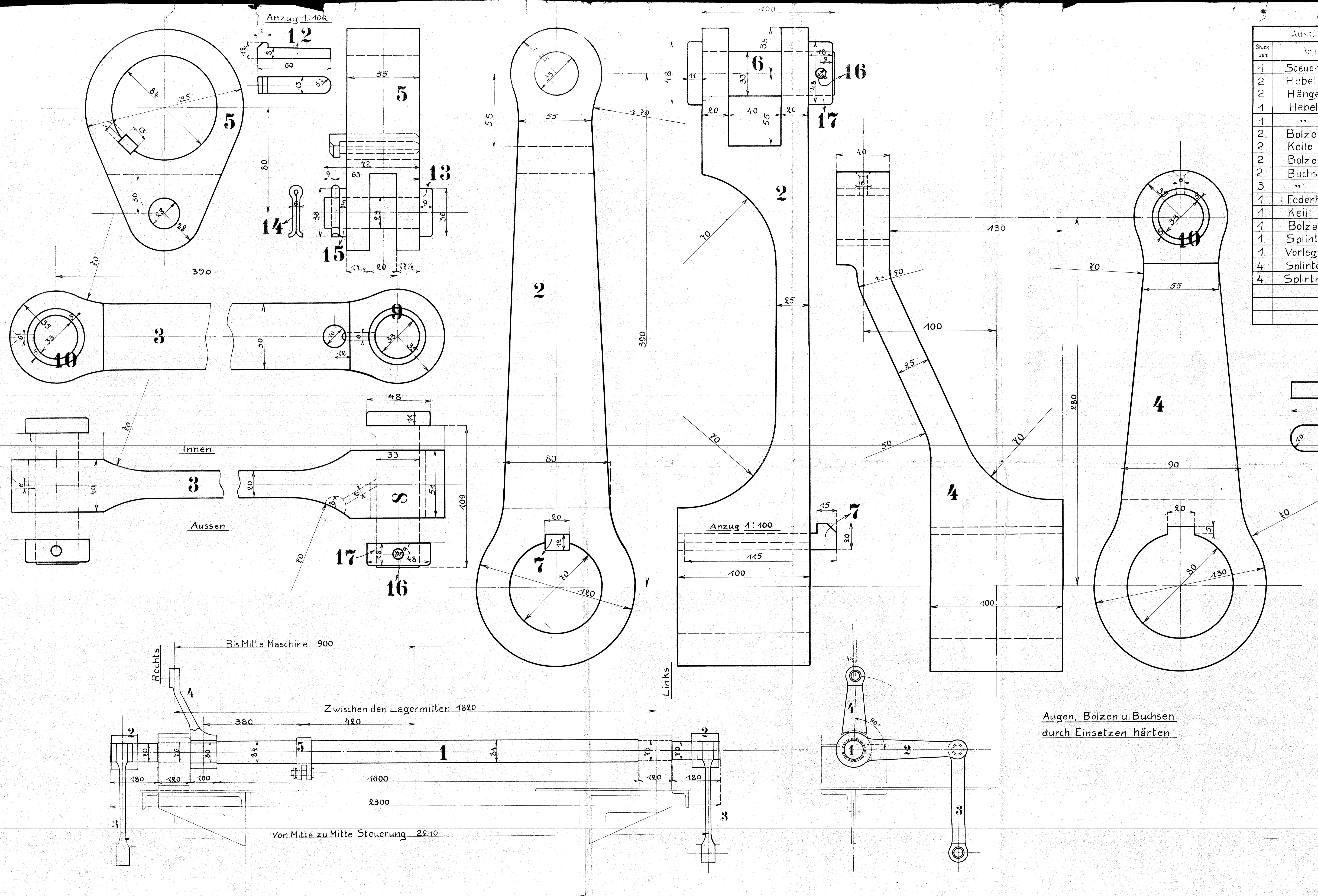
Steuerwelle mit Hebeln.
