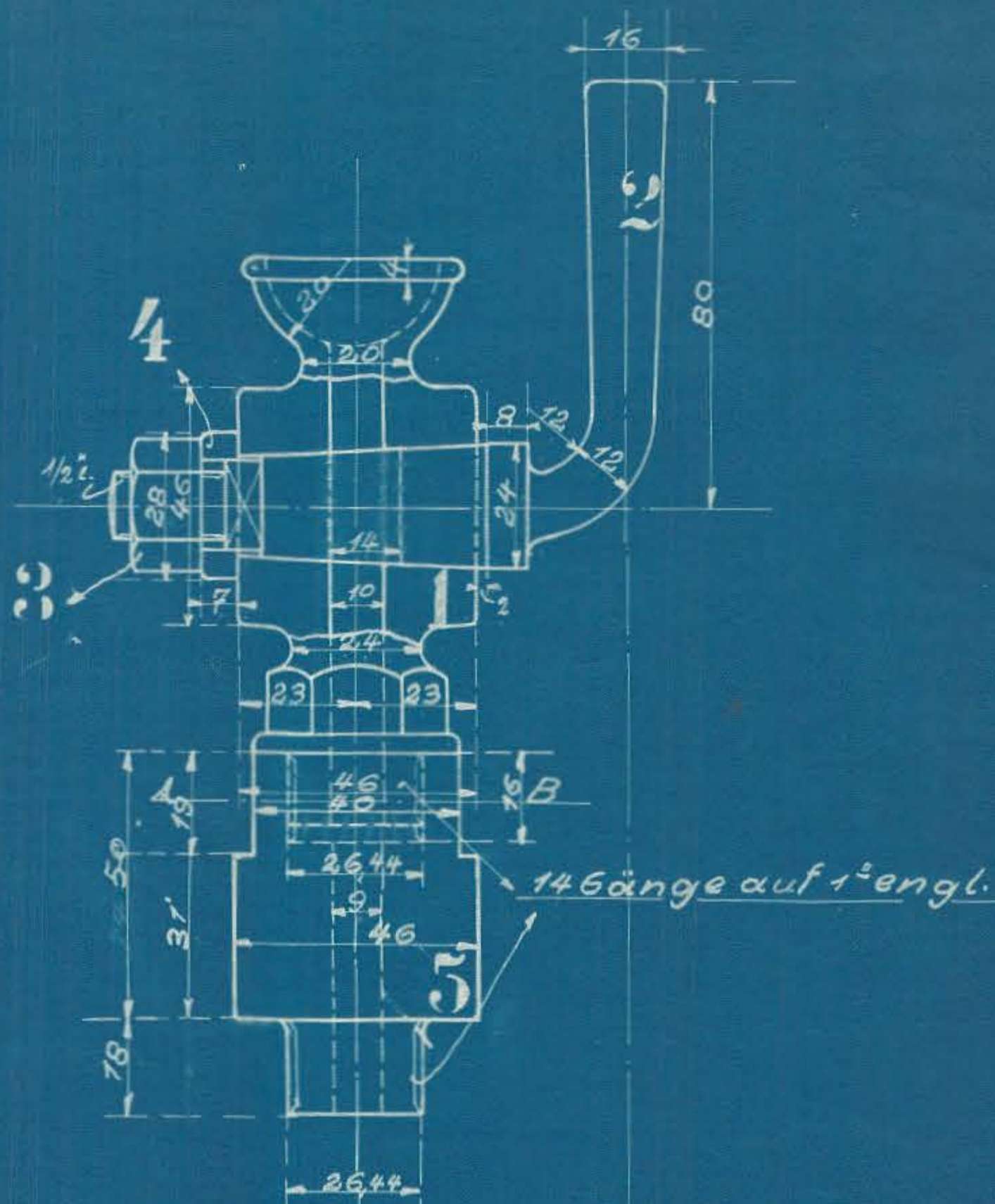
Schnitt A-B
