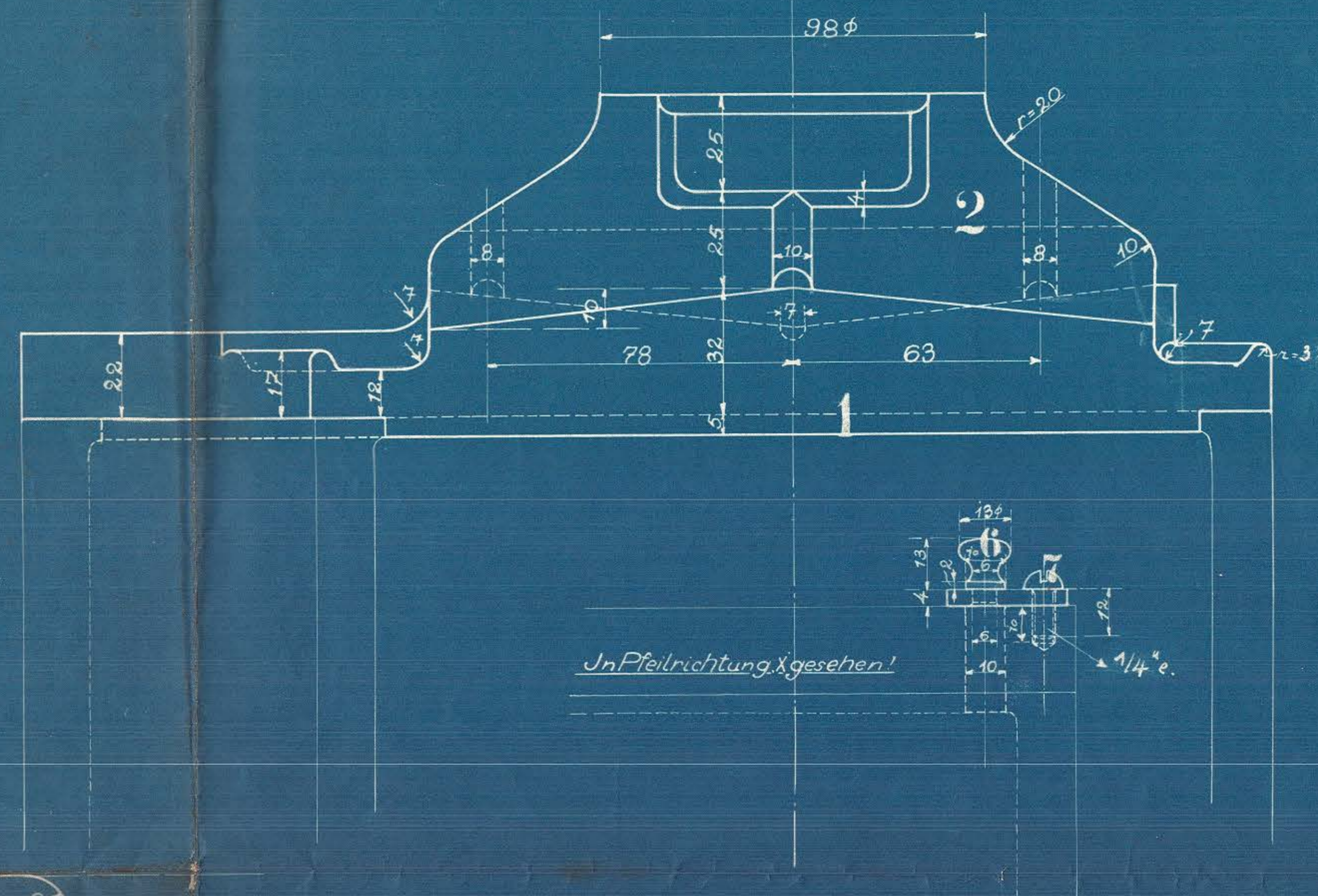
Schnitt C-D
