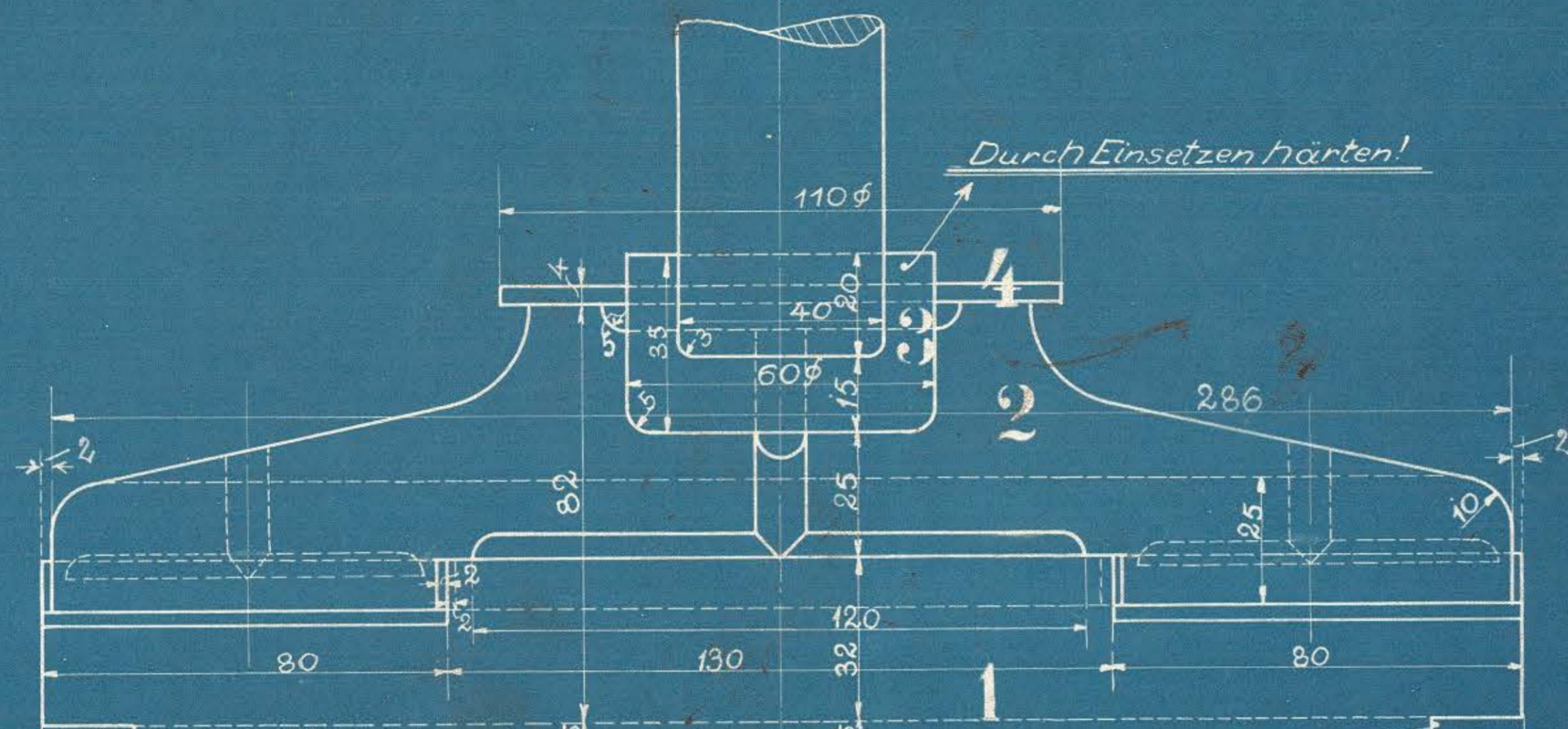
Schnitt A-B
