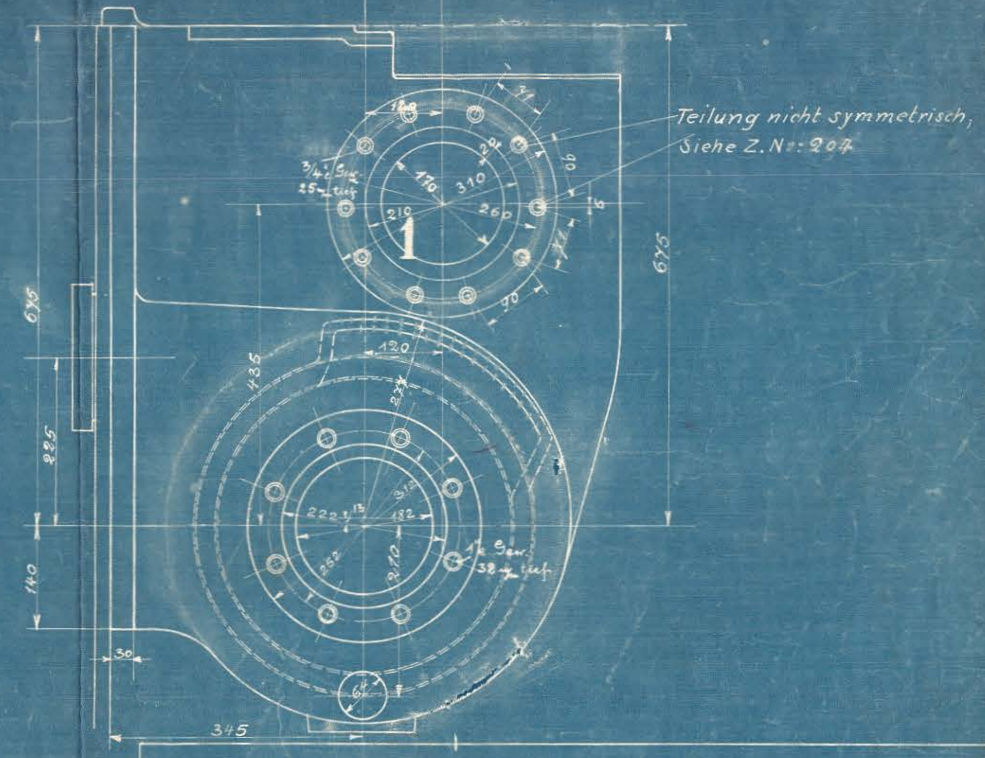
Rechter Cylinder. Von hinten gesehen.
