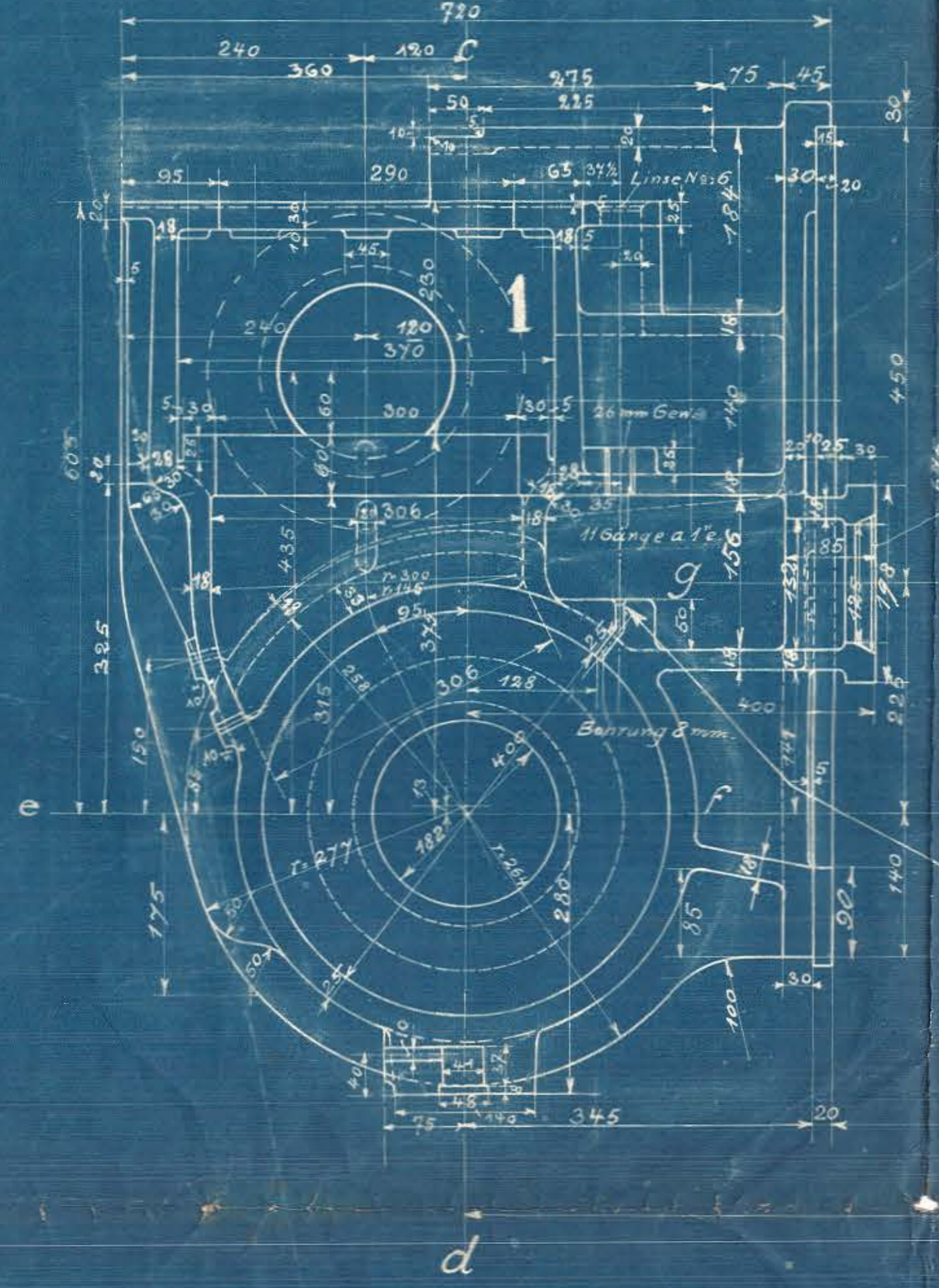
Rechter Cylinder. Schnitt a-b.
