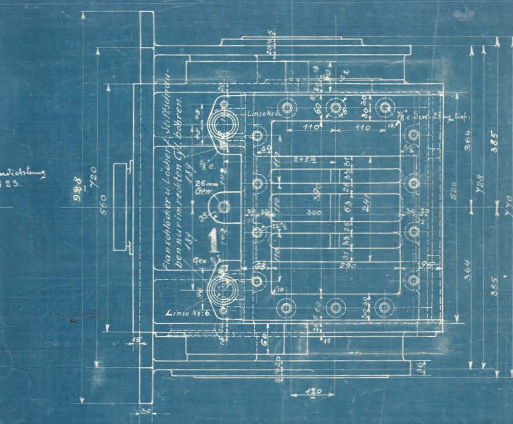
Linker Cylinder. Von oben gesehen.
