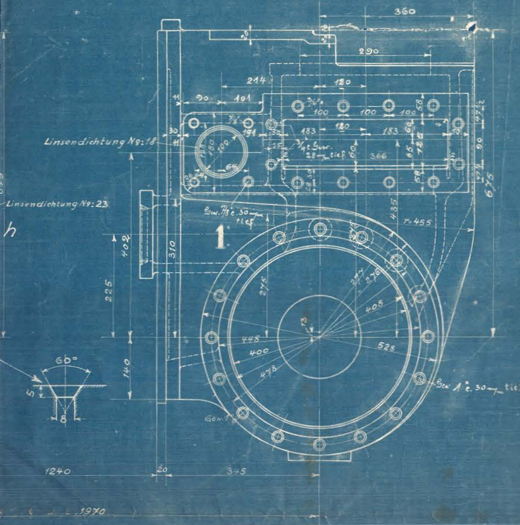
Linker Cylinder. Von vorn gesehen.
