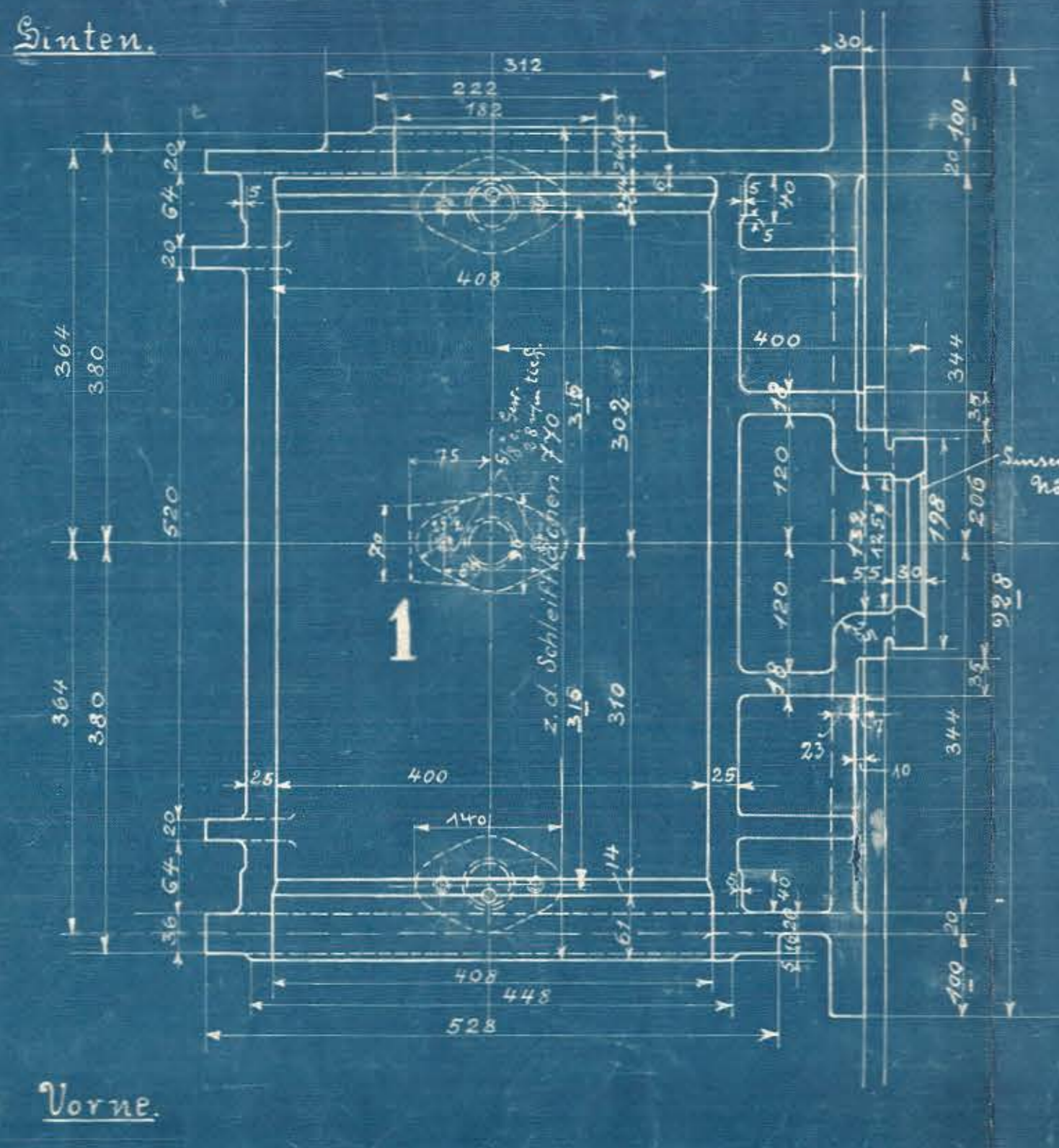
Rechter Cylinder. Schnitt e-f-g-h.
