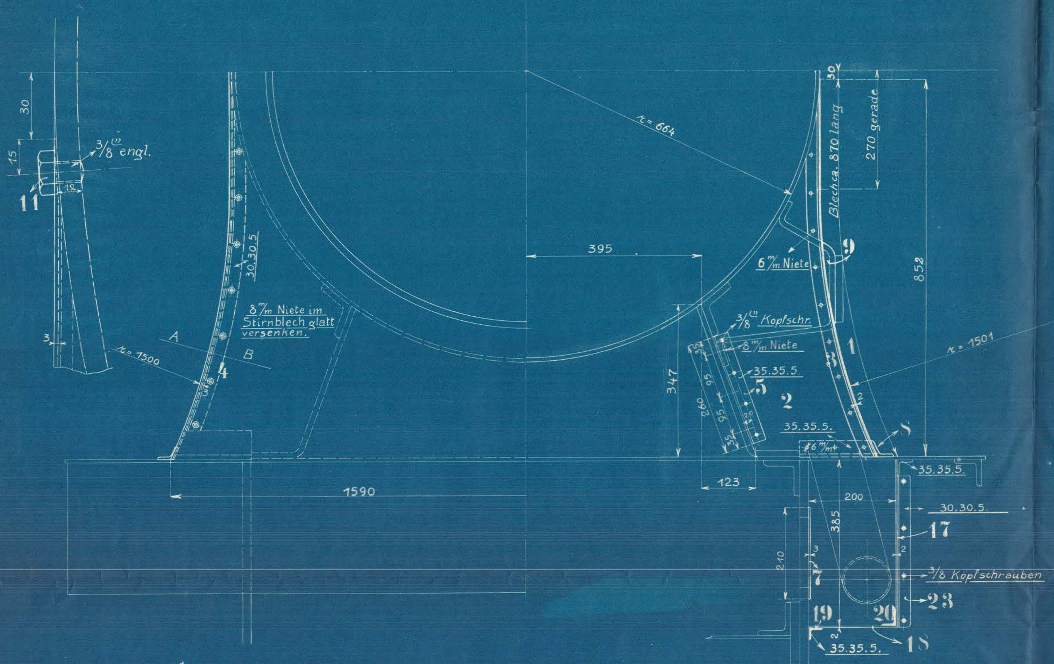
Schnitt A-B.
