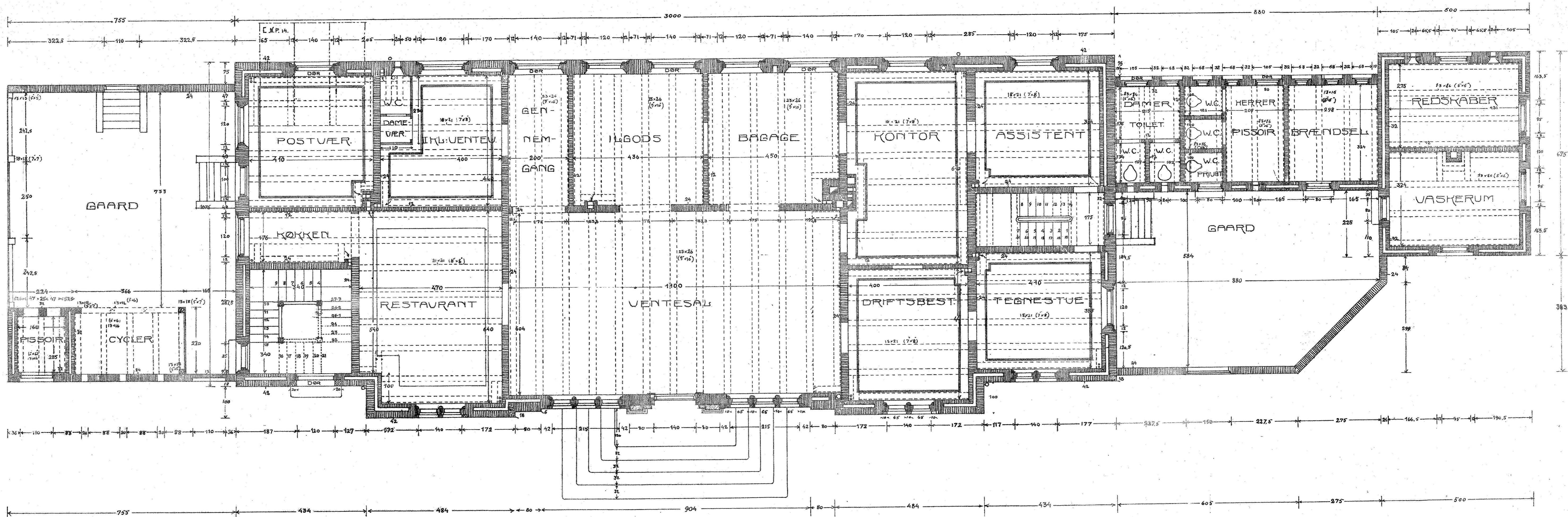
STUEPLAN.
