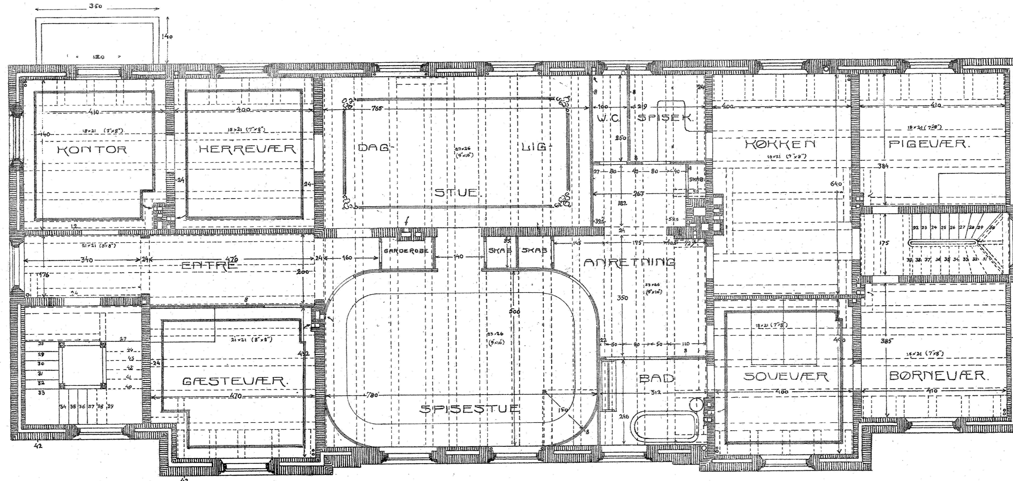
1 STE SALSPLAN.
