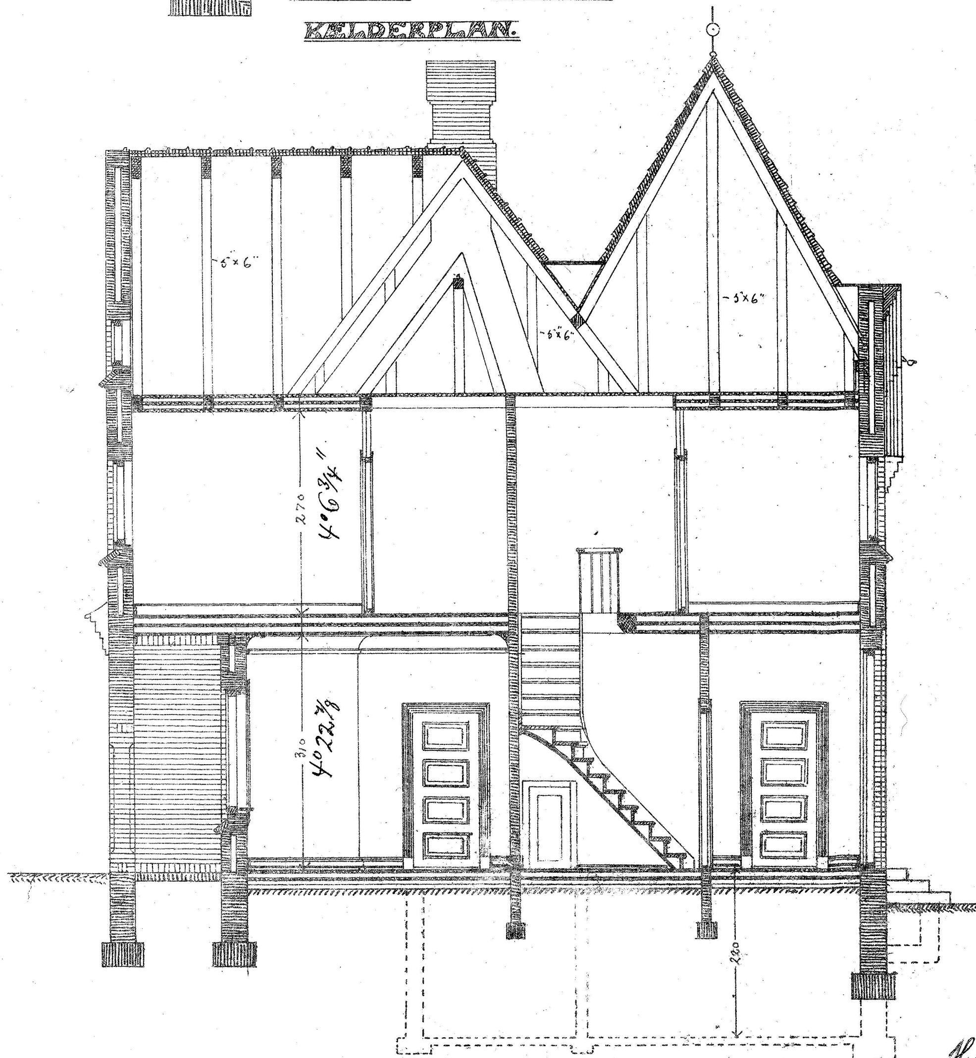
SNIT.
