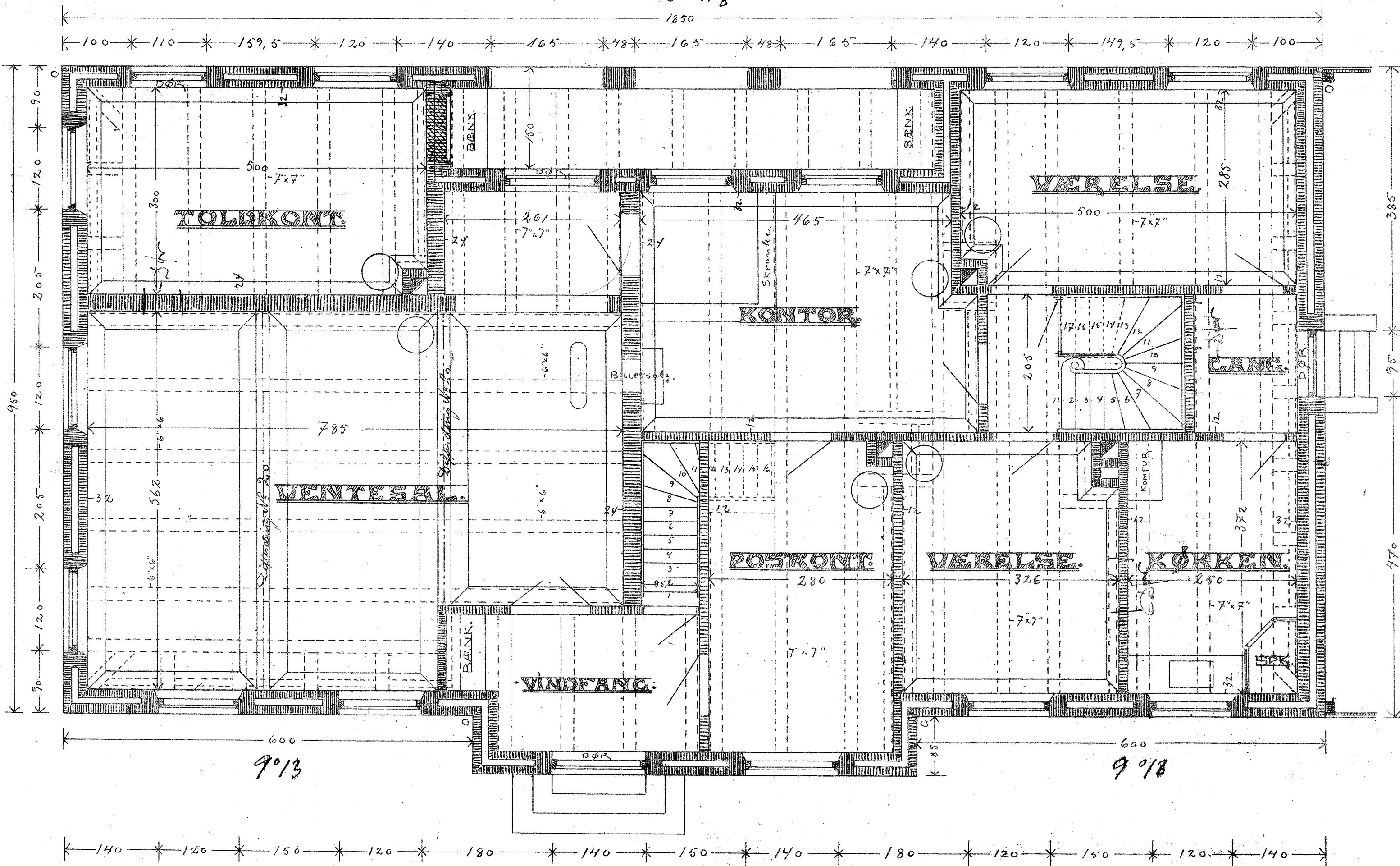
STUEPLAN.
