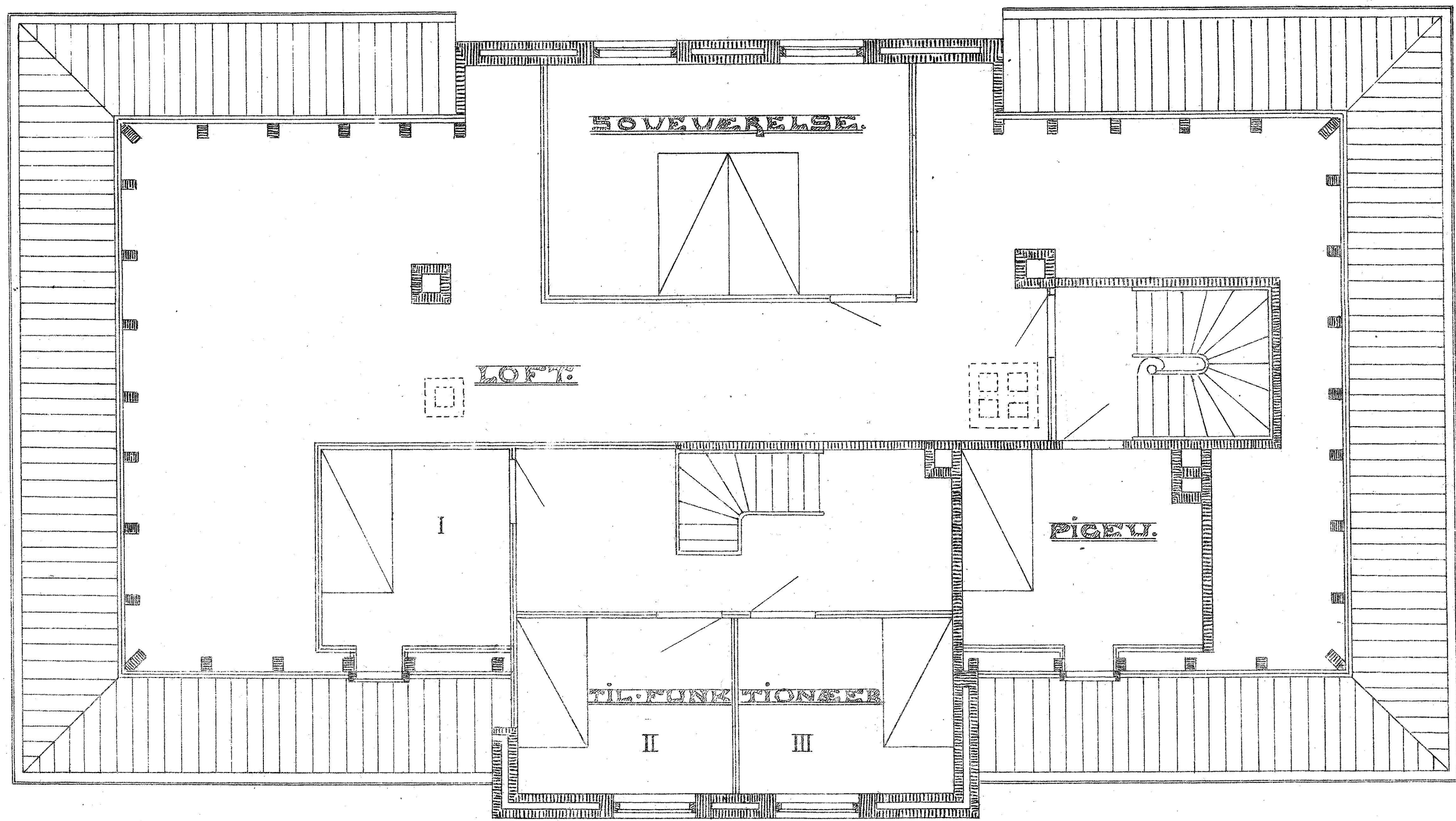
LOFTSPLAN.
