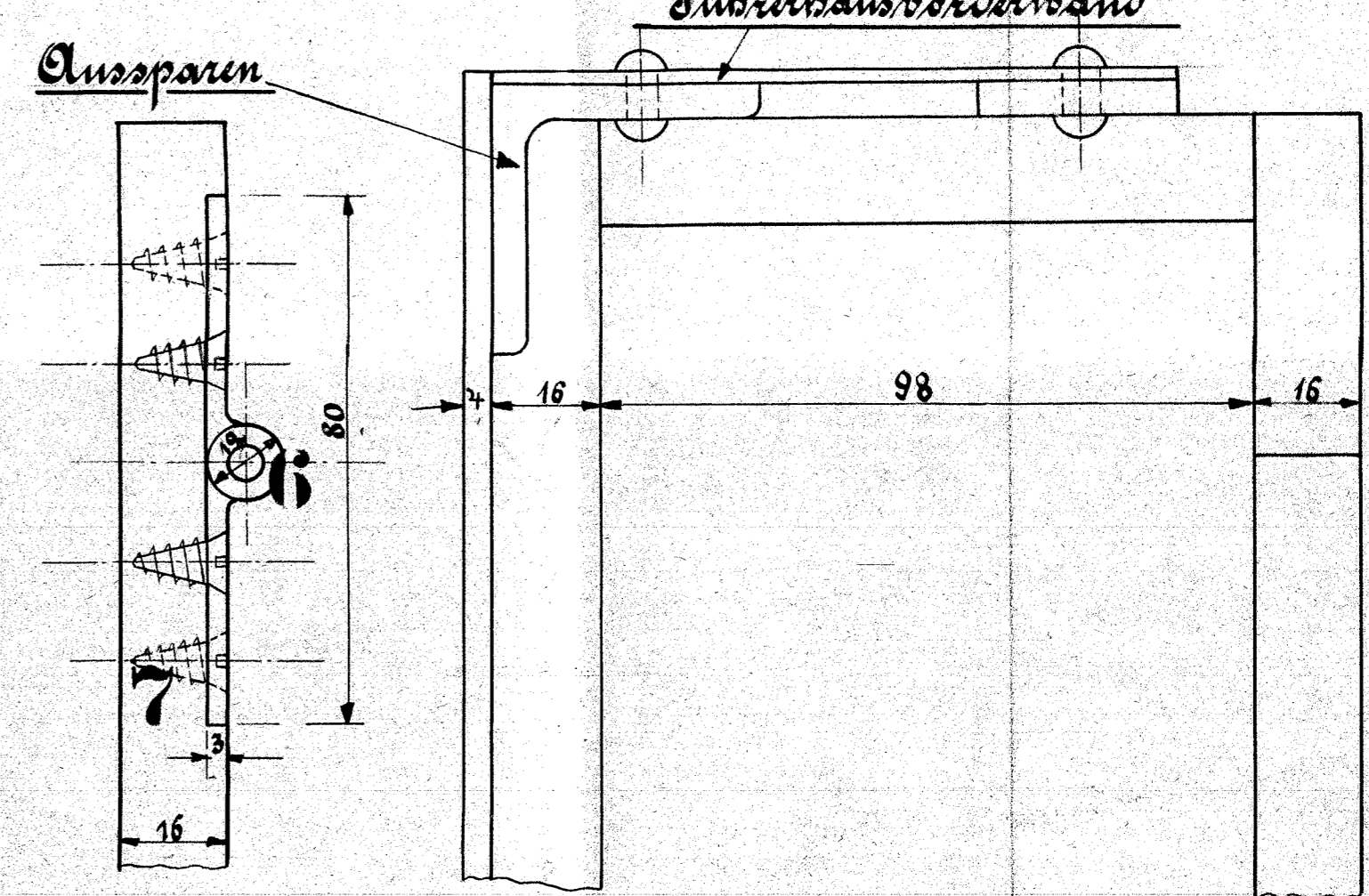
Schnitt A-B
