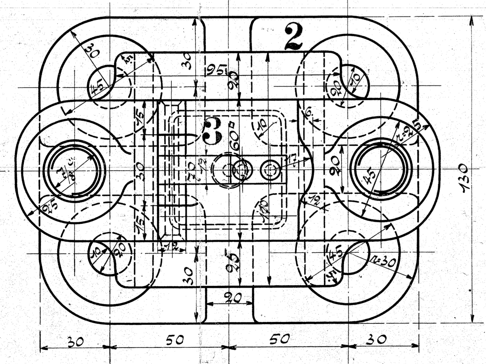
Schrauben & Muttern nach dänischer Tabelle.
