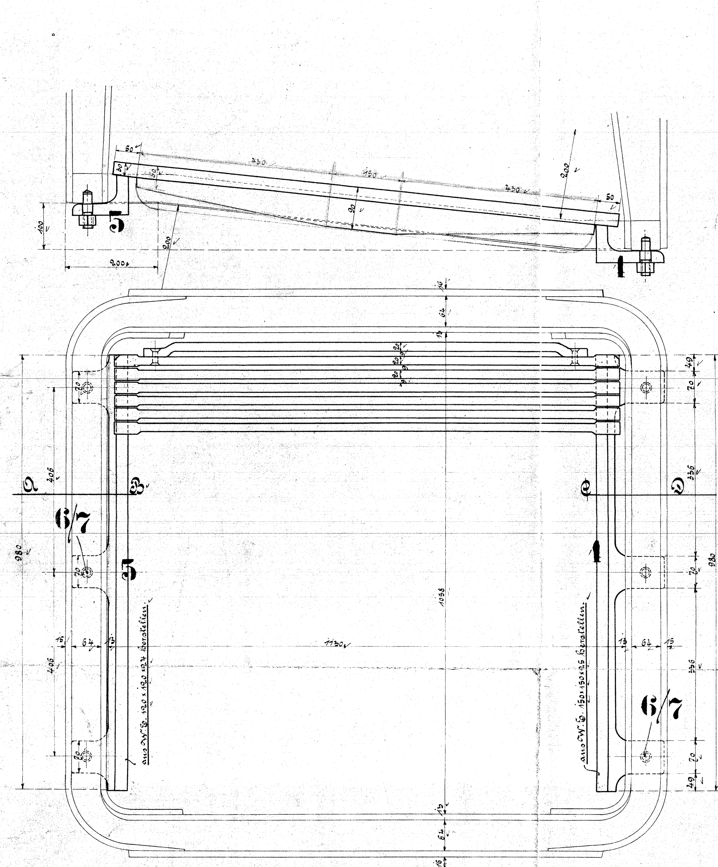
Schnitt A-B
