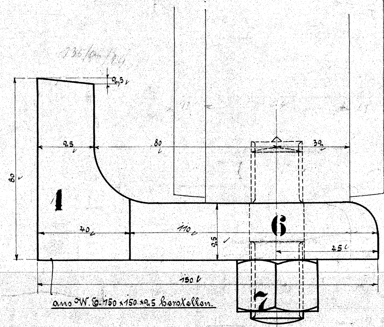
Schnitt C-D
