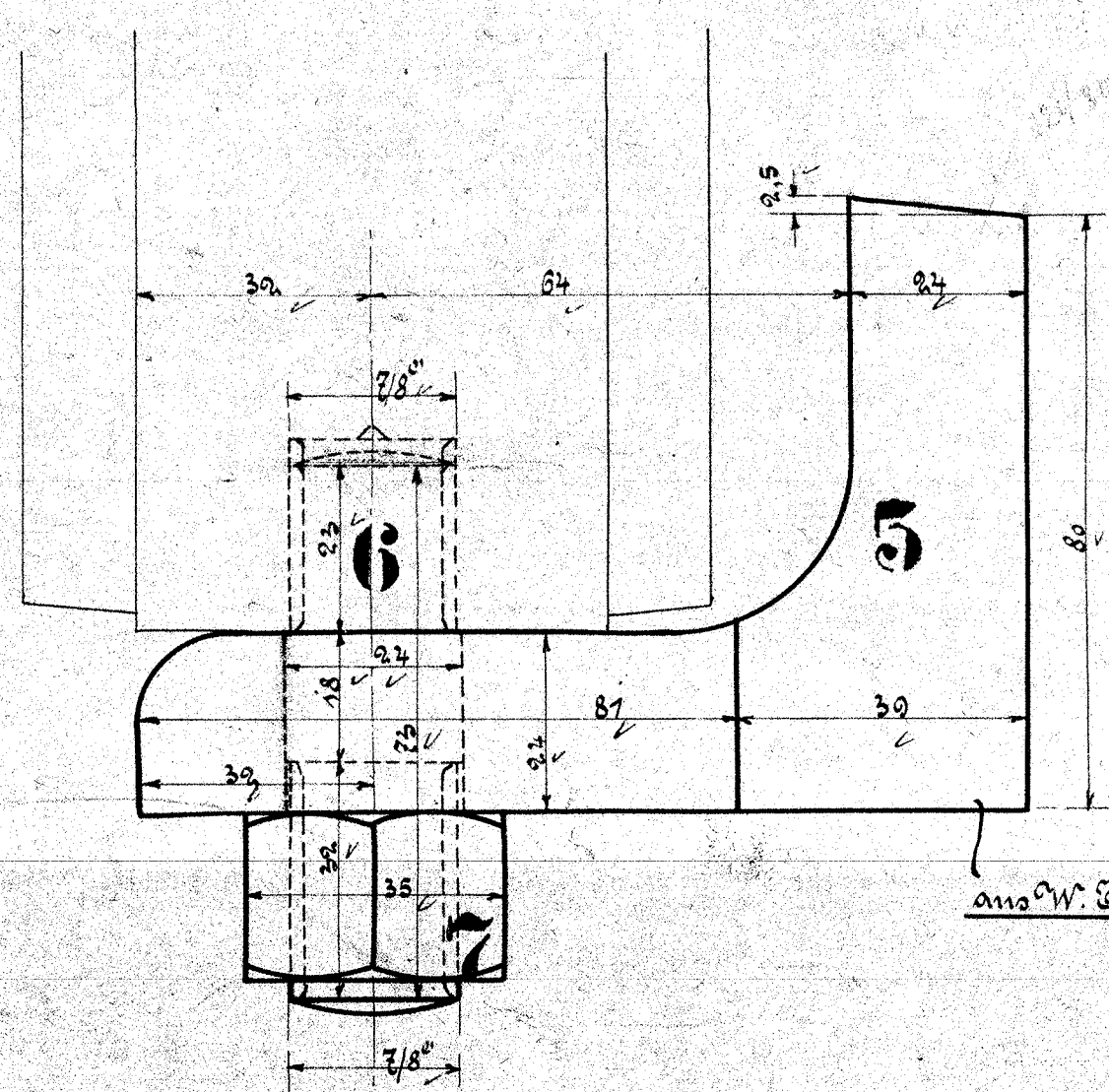
Schnitt A-B
