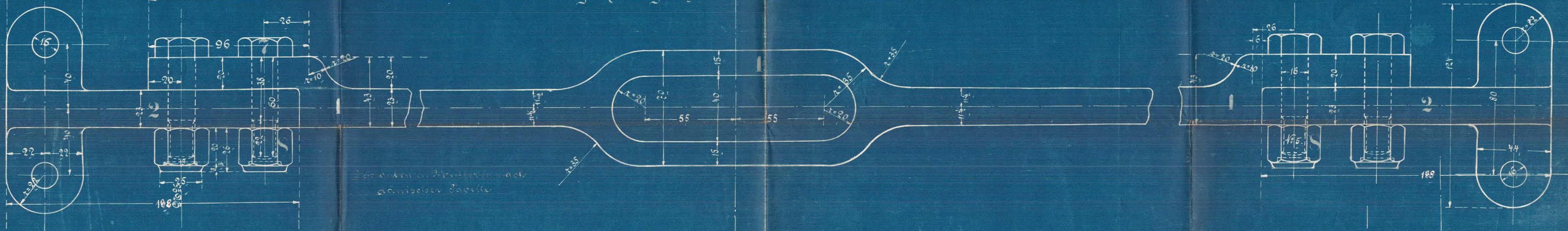
Ganze Länge 990
