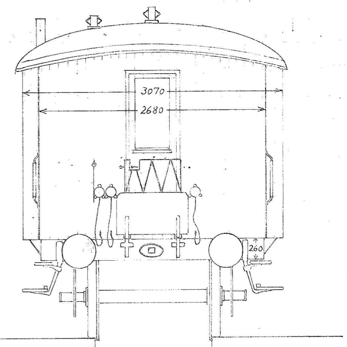
HVJ C 501. Scandia 1920. 28 pl. storrøm + 8 pl. Kupé + post- og rsg.rum. Koksfyr. TB (p), ♀, ♂ → 7,1 m ←, (← 12,87 m →), tara 14,6 t. Opr. HVJ A 501, ren pers., 28 III + 2x8 II, åbne perroner, ingen bremse, men Vacuumledning. 1932 koksfyr (motorlok. anskaffet). 1951 omb. m. luk.perr, polstr.sæder, TB + ♀. Senere er den ene „fine“ kupé omb. til post- og rsg.-rum.
