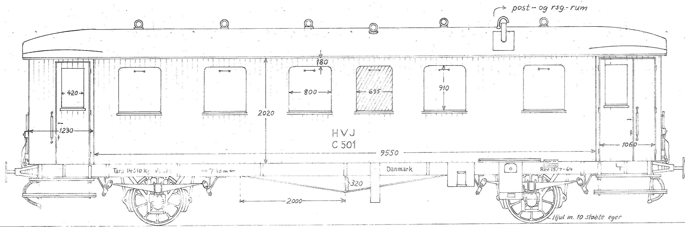
HVJ C 501. Scandia 1920. 28 pl. storrøm + 8 pl. Kupé + post- og rsg.rum. Koksfyr. TB (p), ♀, ♂ → 7,1 m ←, (← 12,87 m →), tara 14,6 t. Opr. HVJ A 501, ren pers., 28 III + 2x8 II, åbne perroner, ingen bremse, men Vacuumledning. 1932 koksfyr (motorlok. anskaffet). 1951 omb. m. luk.perr, polstr.sæder, TB + ♀. Senere er den ene „fine“ kupé omb. til post- og rsg.-rum.
