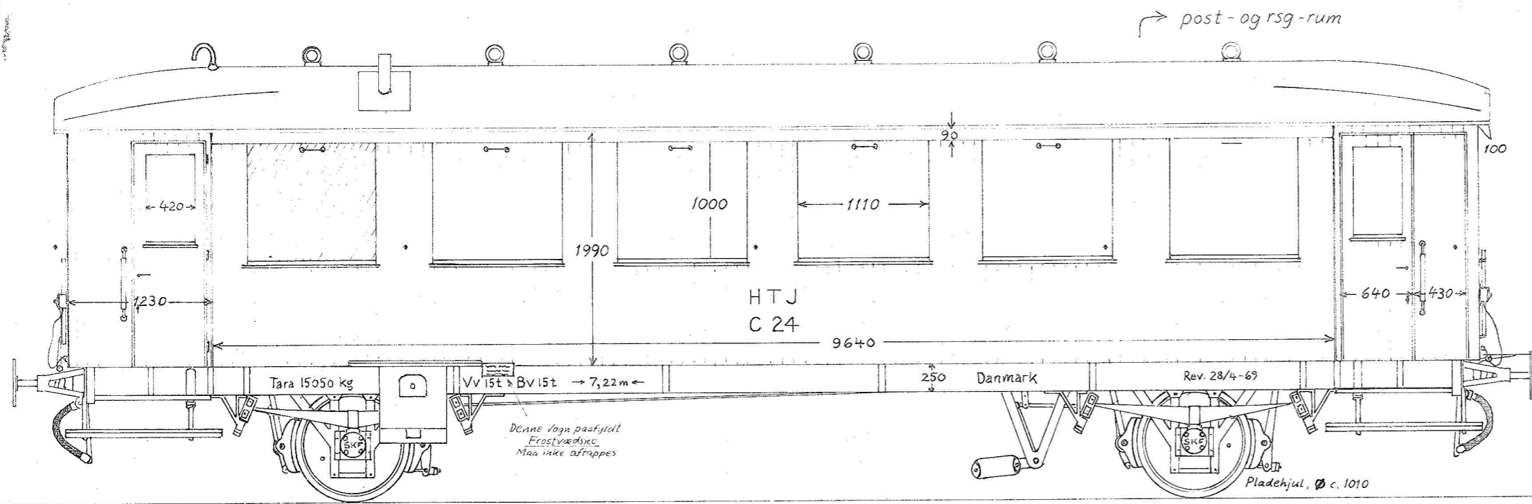
HTJ C 24. Scandia 1911. 46 pl. II kl., post- og rsg.-rum, koksfyr, toilet. TB (p), rullelejer. → 7,22 m ←, (← 13 m →), tara 15 t. Oprind. KS C 2, åbne perroner, ren pers., 56 pl. III kl., toilet, ♀ og ♂ 1949 til HTJ og ombygget. Søstervognene KS C 3, 7 og 9: C 3 → HTJ C 25, ej omb. C 7 og 9 til OHJ C 204/205, sammenbygget på 3 bogier, åbne perroner bevaret i de frie ender, men lukkede perroner m. harmonika i midten, hvor toiletenderne mødes.
