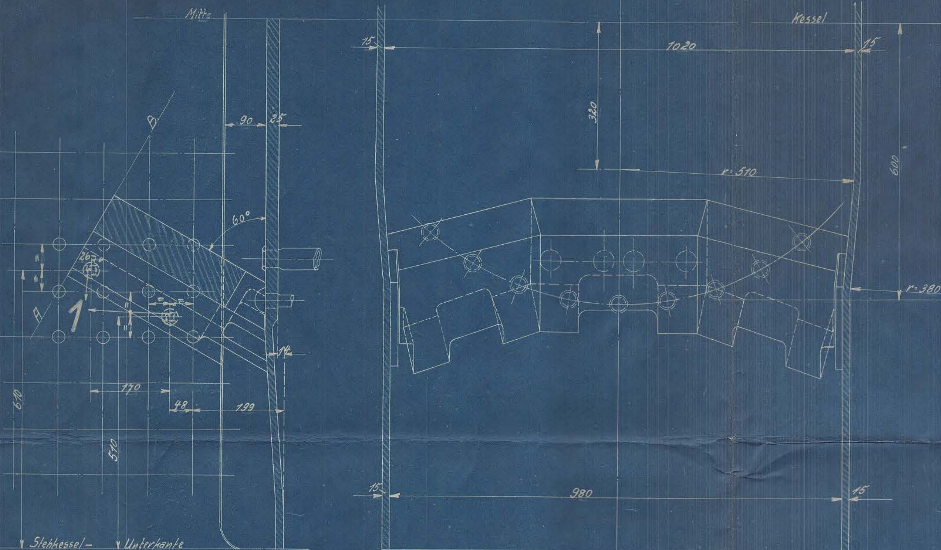
Schnitt A-B
