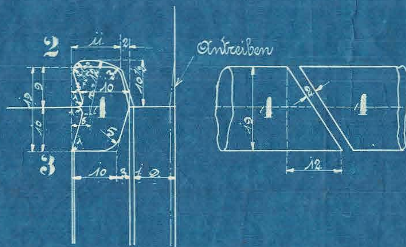
Bandagen Befestigung Derselbe Größe
