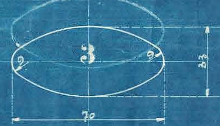
Speichenquerschnitt am Unterteil
