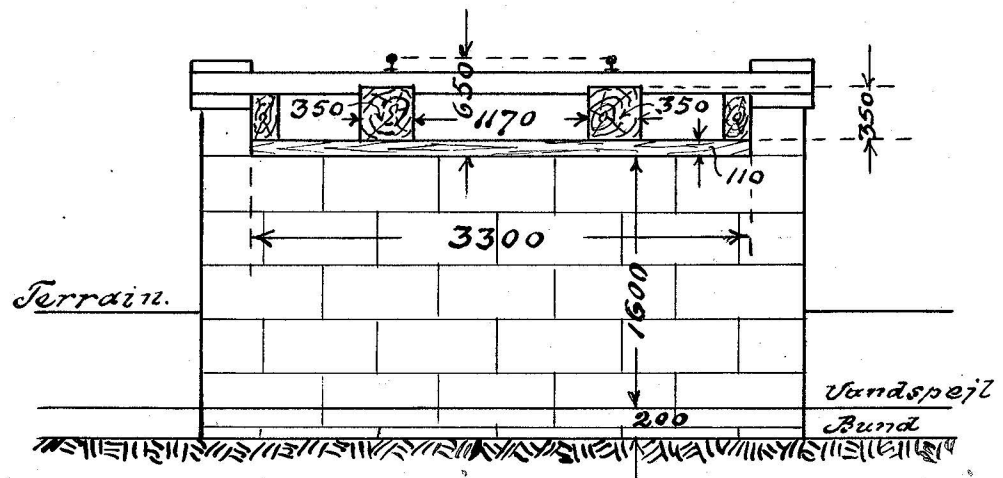
Tværsnit.
