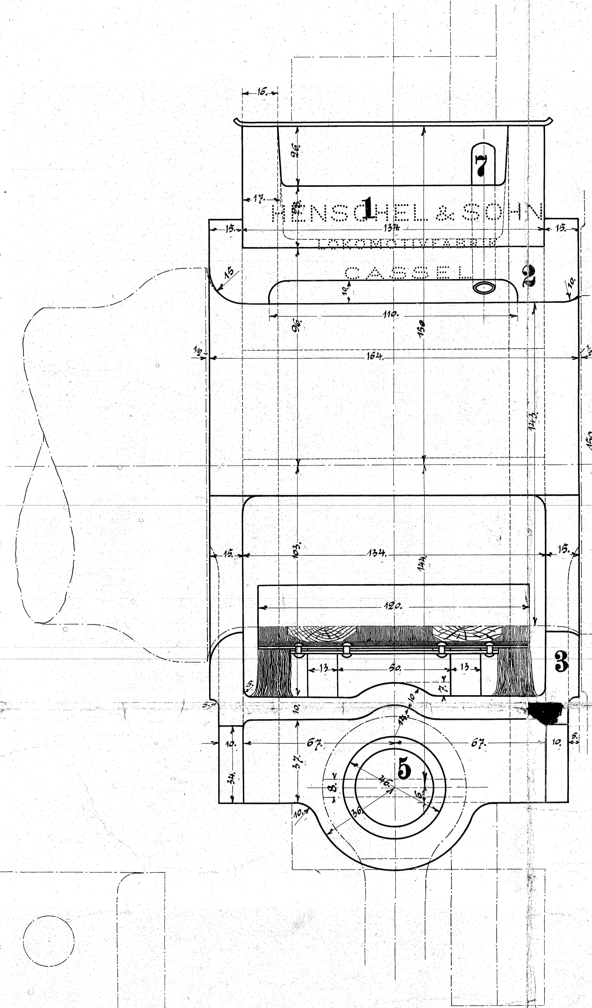
Anführung für eine Lokomotive.
