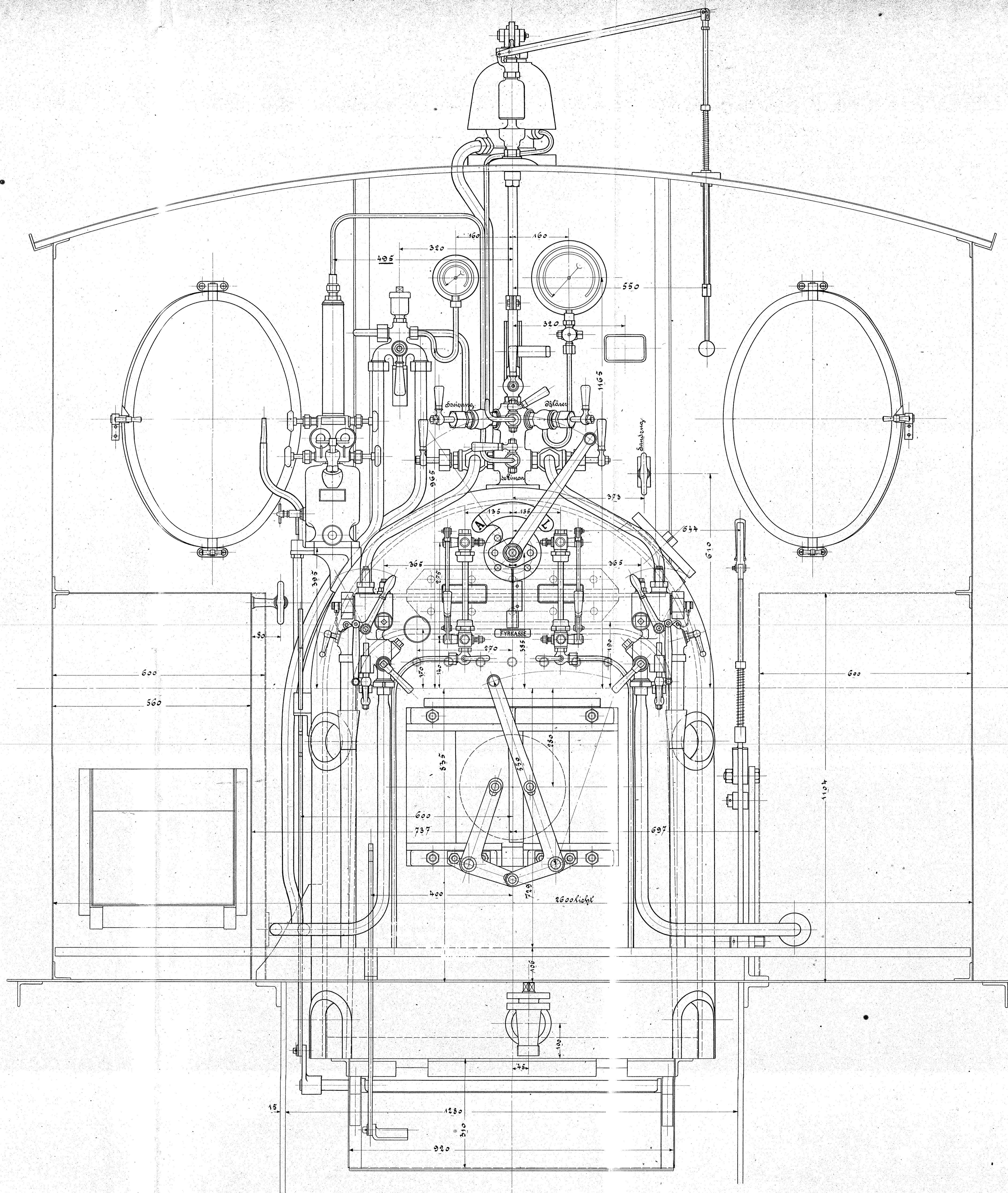
\frac{3}{4} geh. Tender-Lokomotive für die Soersingör-Boornbach-Bahn. Fabr. No: 2525.
