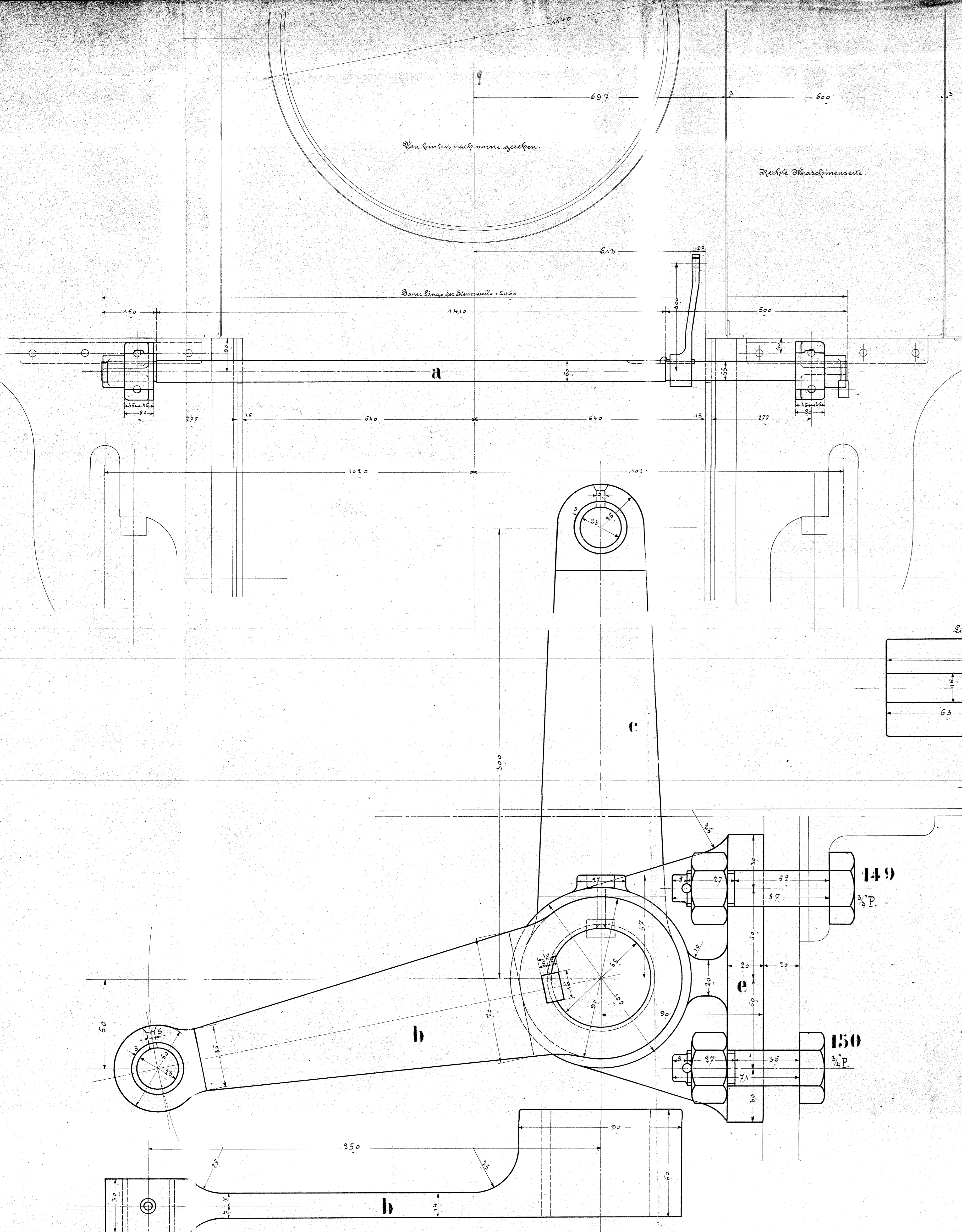
Steuerschwelle mit Lagern.
