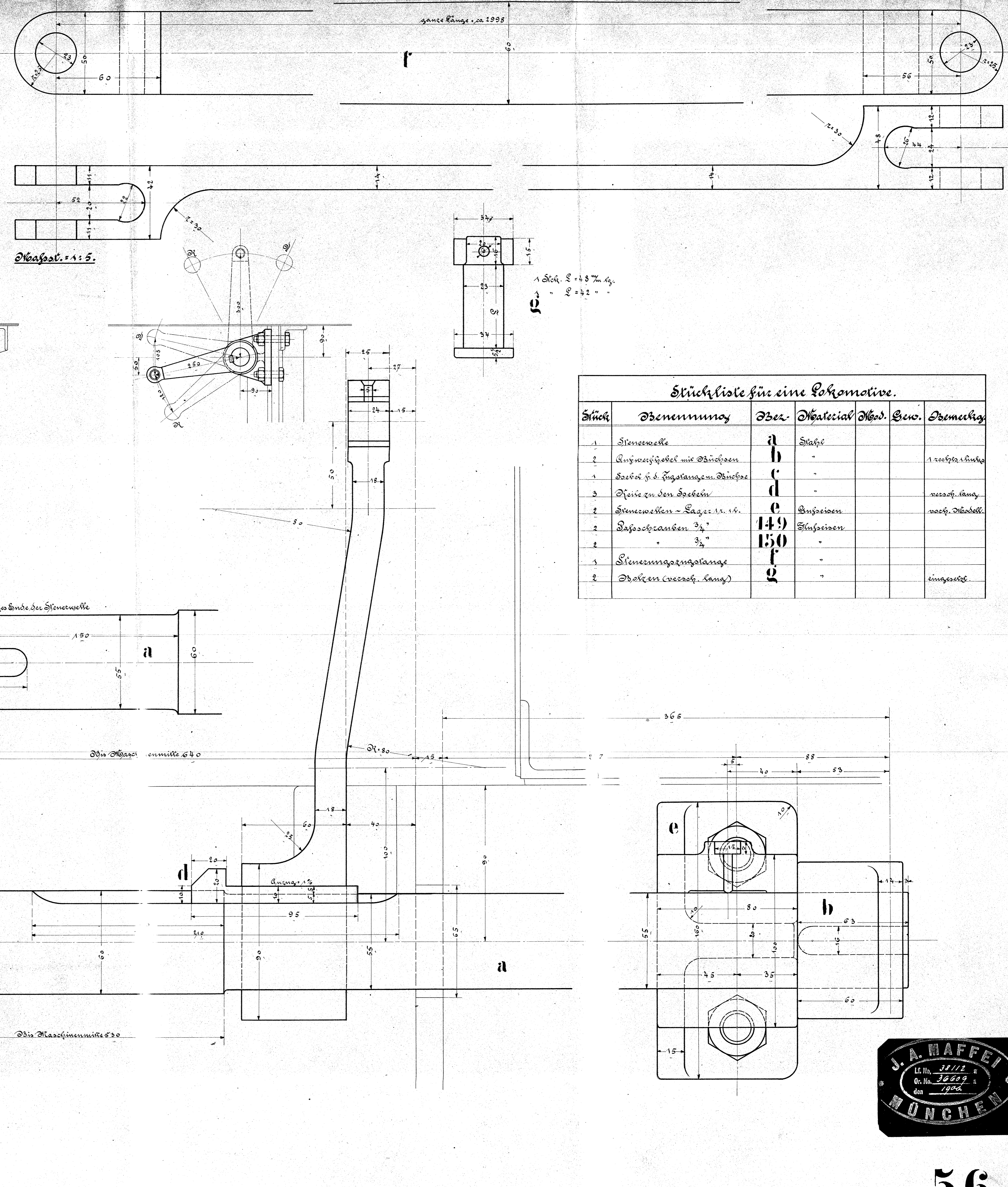
3/4 gch. Tender-Lokomotive für die Sächsisch-Böhmer-Bahn. Fabr. Nr. 2525.
