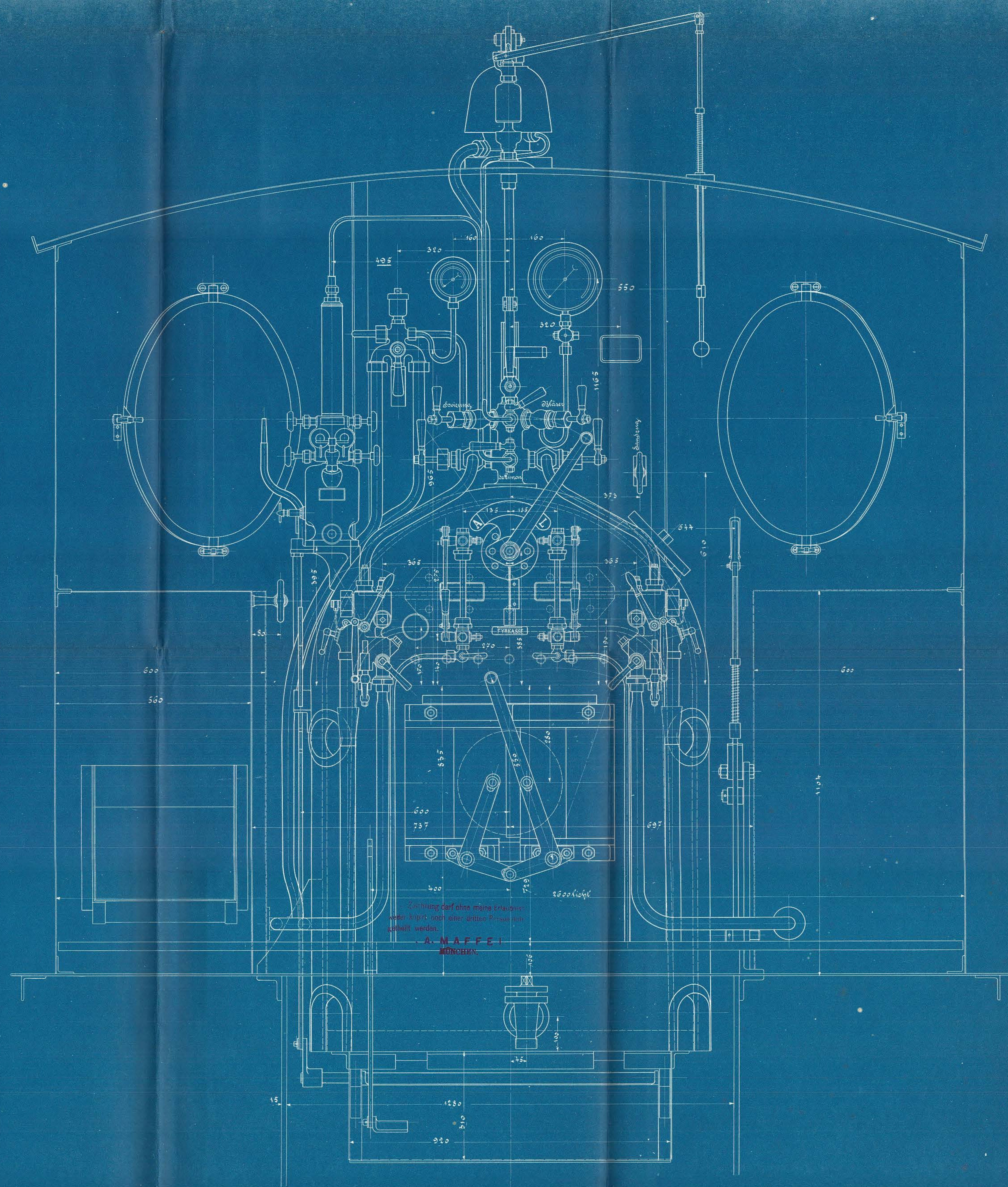
2/3 gek. Tender-Lokomotive für die Soelsingör-Doornbach-Bahn. Fabr. Nr. 2525.
