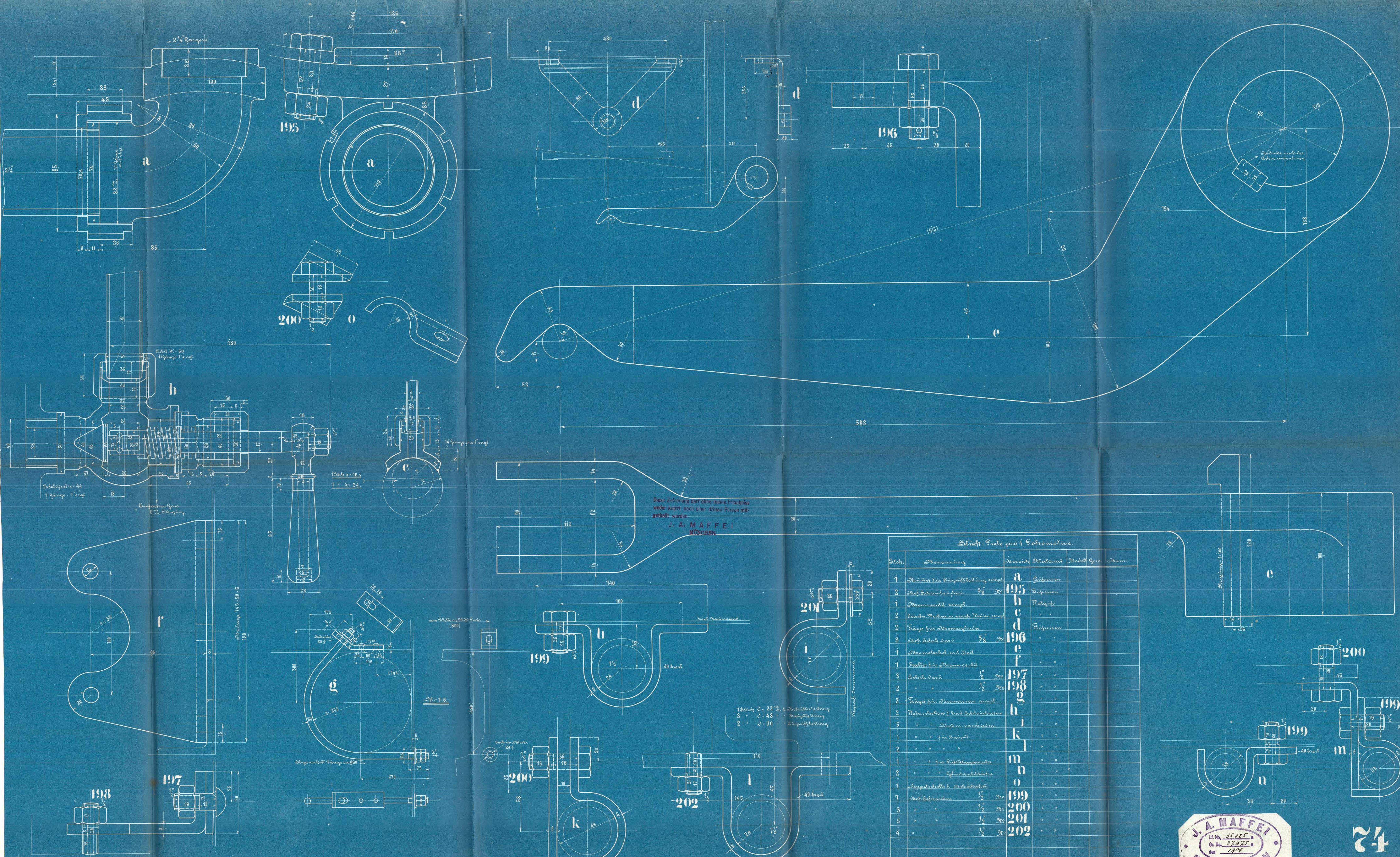
Sicherheitsbremse-Details.
